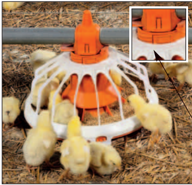
FLUXX 360 met platte gegolfde pan, afsluitschuif en rooster met 16 verdelingen
