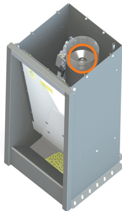
Klapna valova otvorena – male porcije hrane se ispuštaju u valov –
