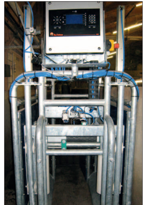
Eine Rolle von oben simuliert die Brust des Ebers im aufgesprungenen Zustand
