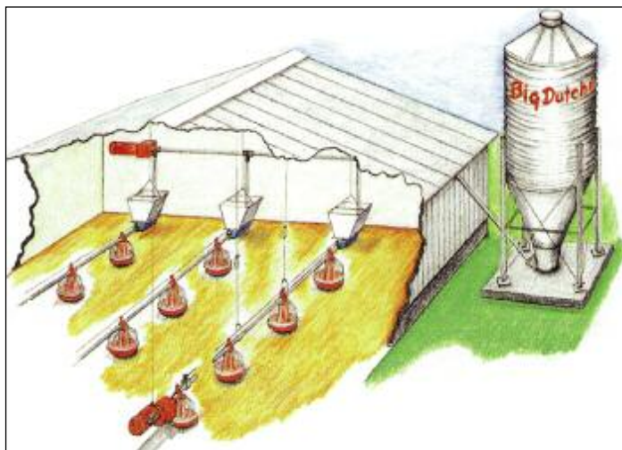
Schématické znázornění stáje s liniemi AUGERMATIC
