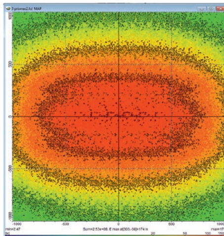
Распределение света с отражателем
