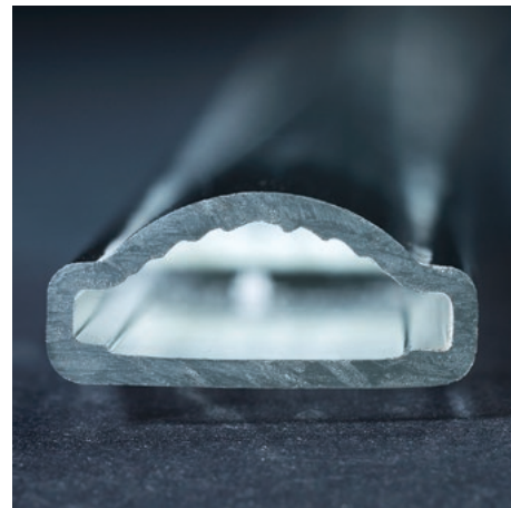
Специальный профиль представляет собой сочетание корпуса и отражателя
