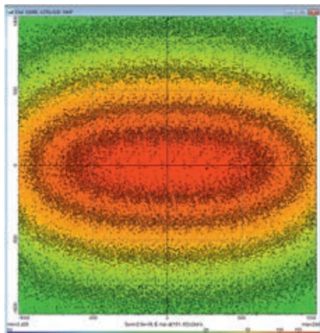
Rozprowadzenie światła bez reflektora
