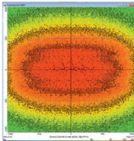
Lichtverdeling met reflector
