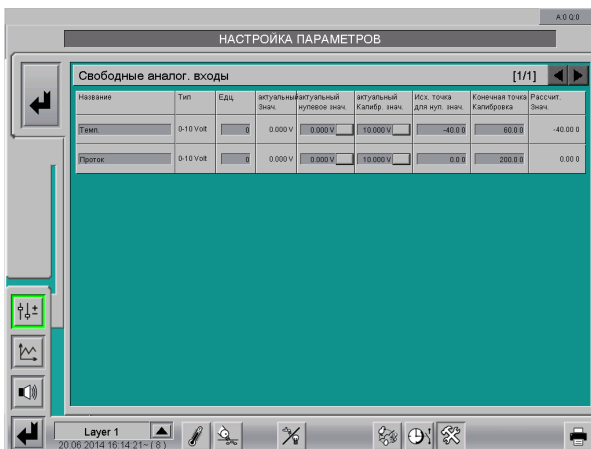
Рис. 9-9: Настройка свободных аналоговых входов
