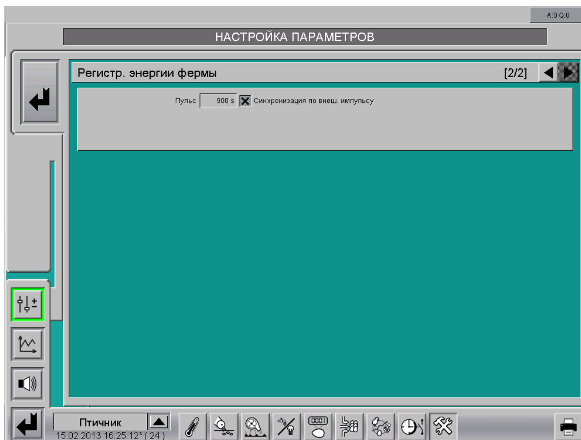
Рис. 9-24: Настройка "Счётчик энергии фермы"
