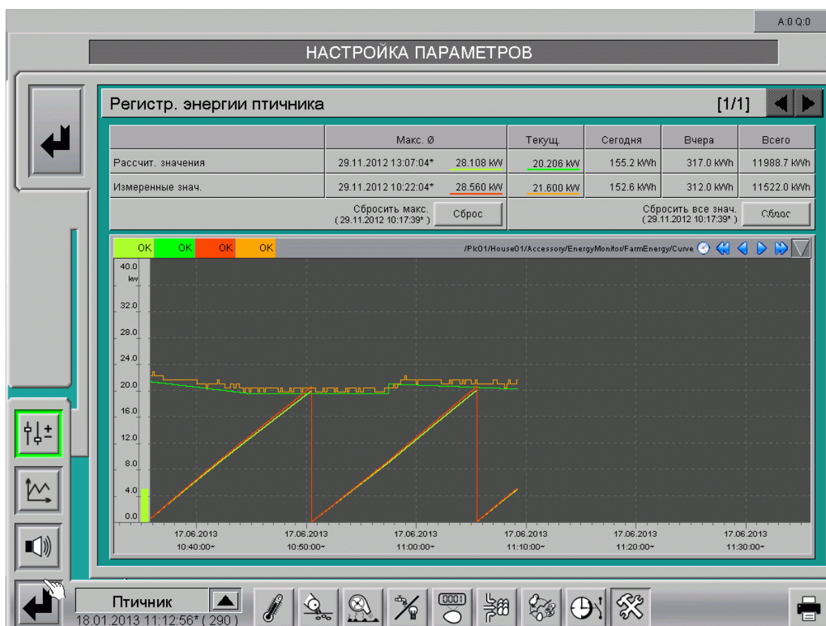
Рис. 9-11: Настройка "Регистрация энергии птичника"
