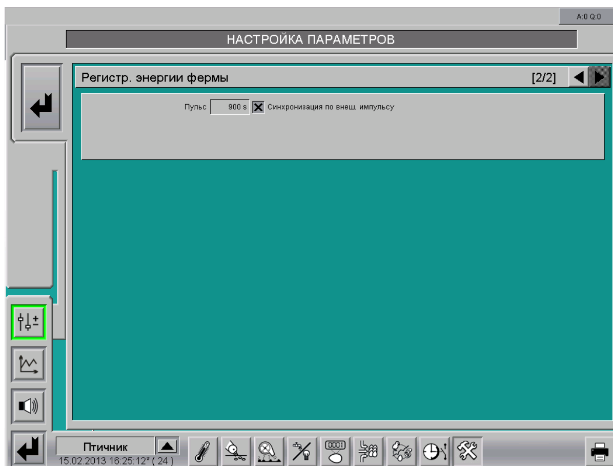
Рис. 9-22: Меню "Регистрация энергии фермы"
