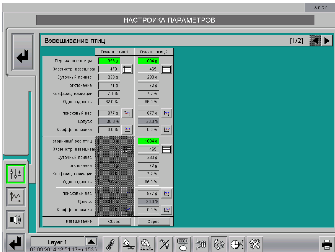
Рис. 7-3: Данные весов для птиц в виде обзора
