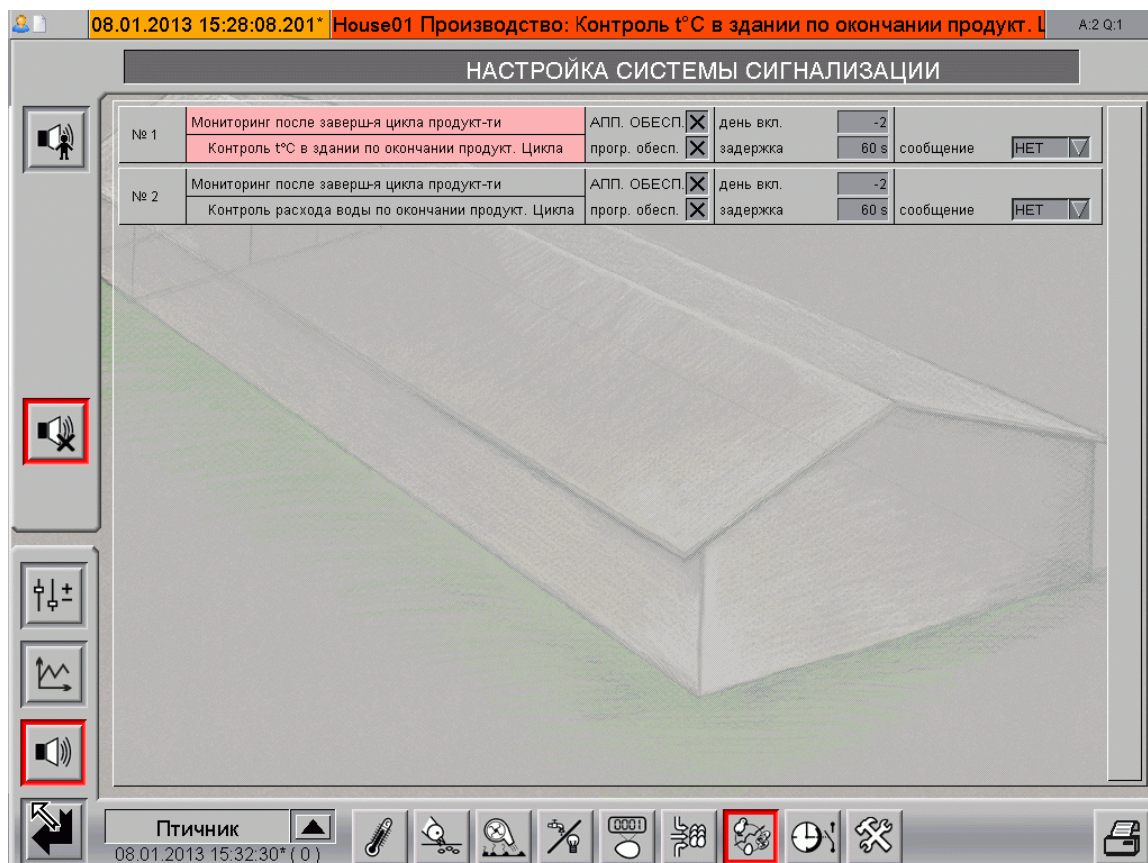
Рис. 11-1: Настройка системы выдачи сигналов тревоги
