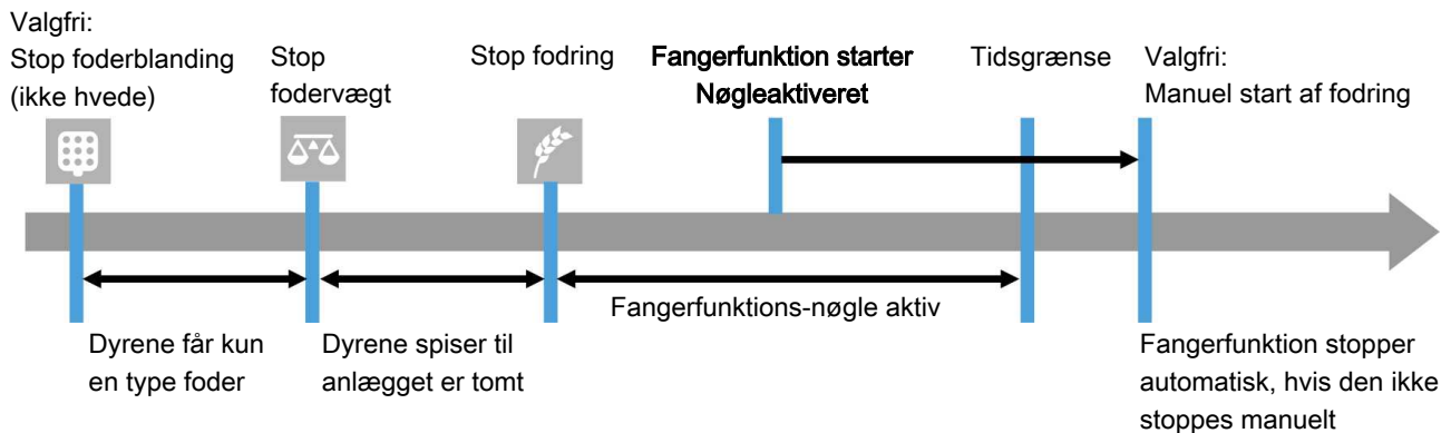
Figur 41: Tidsforløbet ved stop af foderanlæg under fangerfunktion
