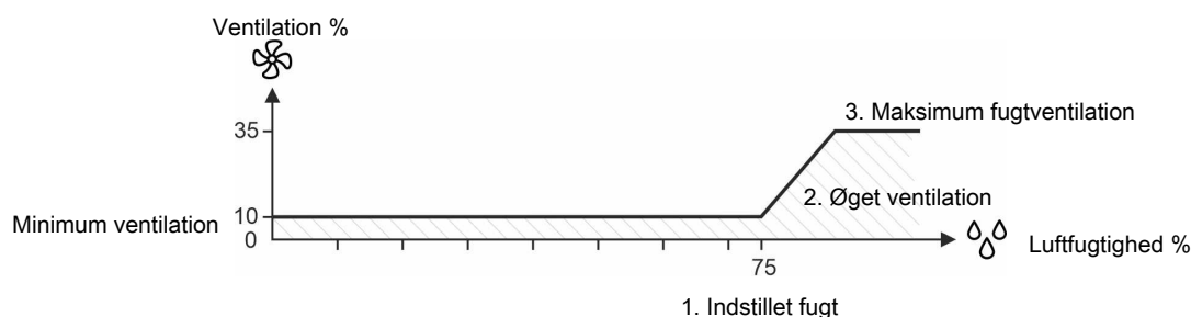
Figur 12: Fugtventilation: 1. Luftfugtigheden overstiger indstillet fugt. 2. Staldcomputeren øger ventilation. 3. Forøgelse op til maksimum fugtventilation (35 %).
