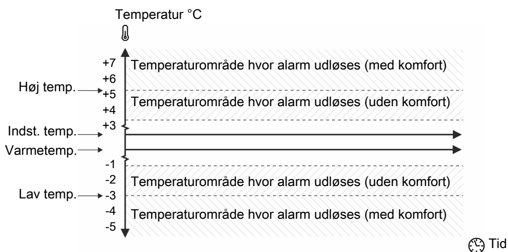
Figur 43: Alarm høj og lav temperatur
