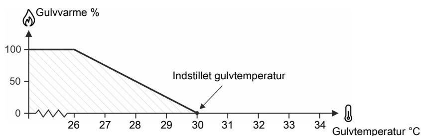
Figur 39: Gulvvarme med temperaturføler
