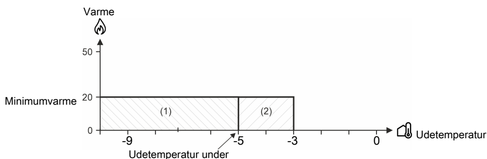
Figur 38: Minimumvarme ved faldende eller stigende udetemperatur
