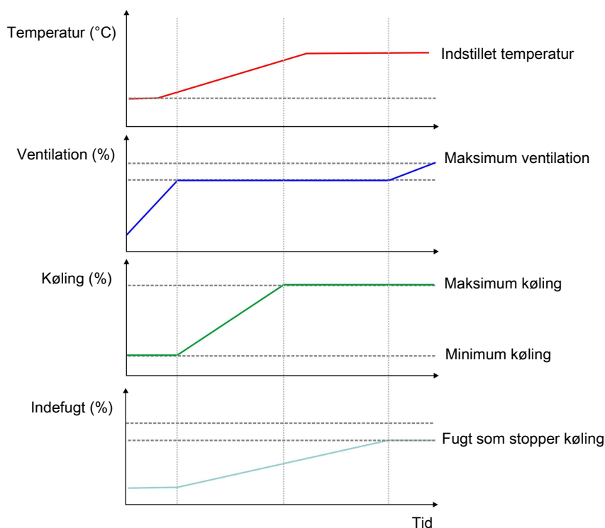
Figur 32: For at holde den ønskede indetemperatur starter kølingen allerede, inden ventilationsniveauet når Maksimum ventilation. Når kølingen ikke kan holde temperaturen, øges ventilationen igen.
