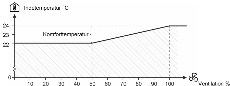
Figur 8: Komforttemperatur ved kontinuerlig drift
