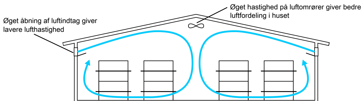
Figur 30: Hus med fritgående dyr hvor ventilationen tilpasses om natten.
