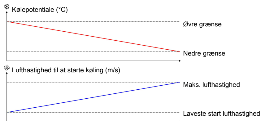
Figur 34: I områder med lav udefugt og et stort kølepotentiale, kan kølingen starte ved en lavere lufthastighed. Omvendt vil man i områder med lavt kølepotentiale vente så længe som muligt med at starte kølingen, så den starter ved maksimum lufthastighed.
