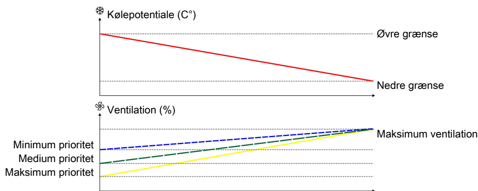
Figur 33: Jo højere kølepotentiale, desto højere prioritet på tidlig start af køling.
