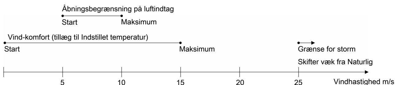
Figur 27: Naturlig ventilation ved stigende vindhastigheder
