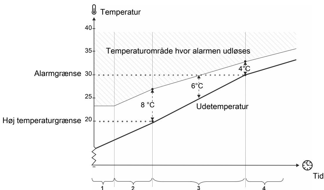
Figur 44: Sommertemperatur ved 20 °C og 30 °C ude
