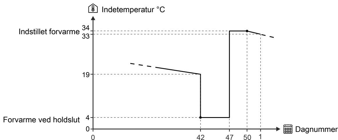
Figur 42: Eksempel på indstilling af forvarme.
