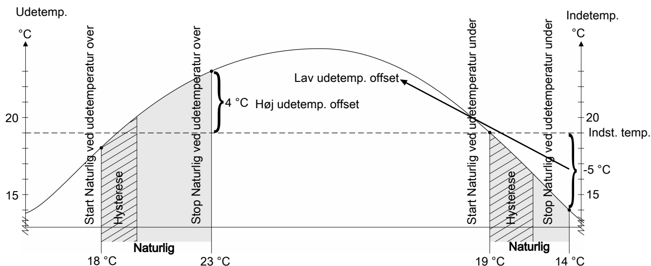
Figur 26: Naturlig ventilation er aktiv afhængig af den aktuelle udetemperatur.
