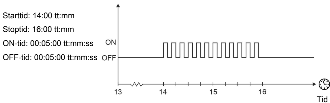
Figur 28: Døgnursregulering
