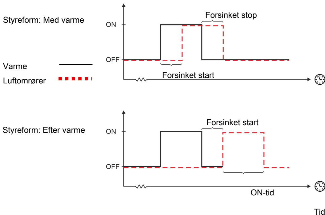
Figur 29: Varmekilderegulering
