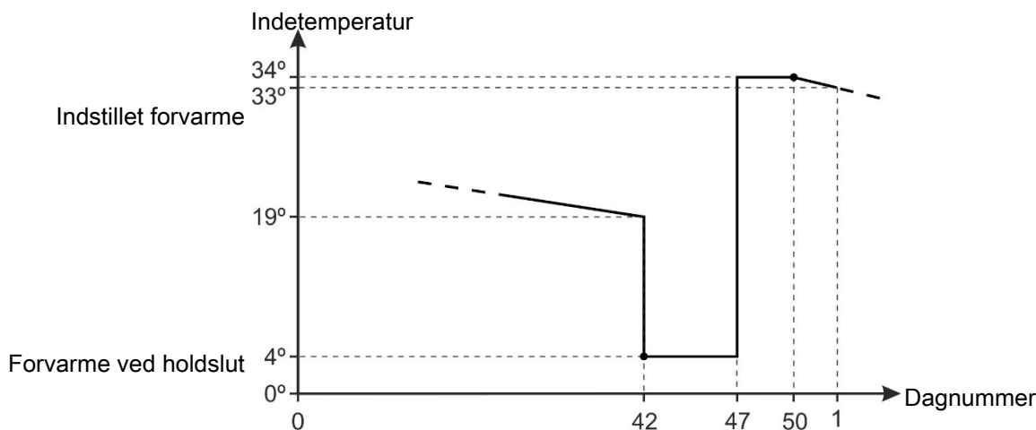
Figur 10: Eksempel på indstilling af forvarme.
