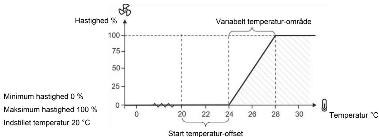
Figur 4: 0-10 V-styret luftomrører med et positivt Start temperatur-offset
