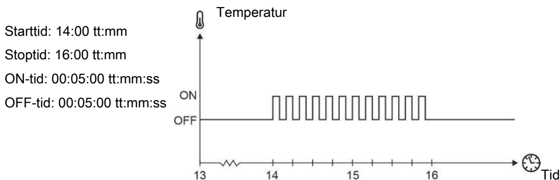
Figur 2: Døgnersregulering
