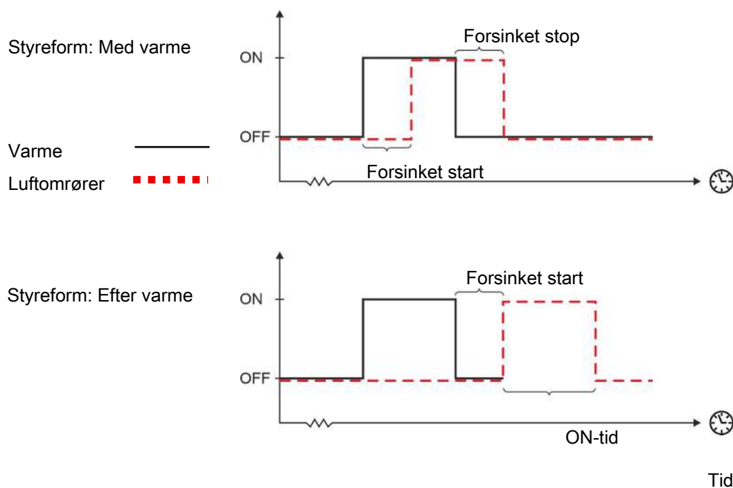
Figur 6: Varmekilderegulering
