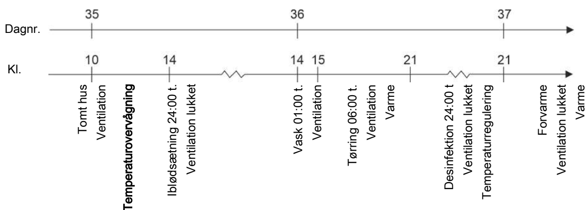
Figur 9: Forløb af Pausefunktioner
