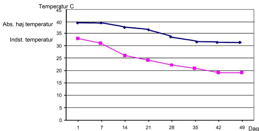
Figur 12: Eksempel på Absolut høj temperatur alarm.
