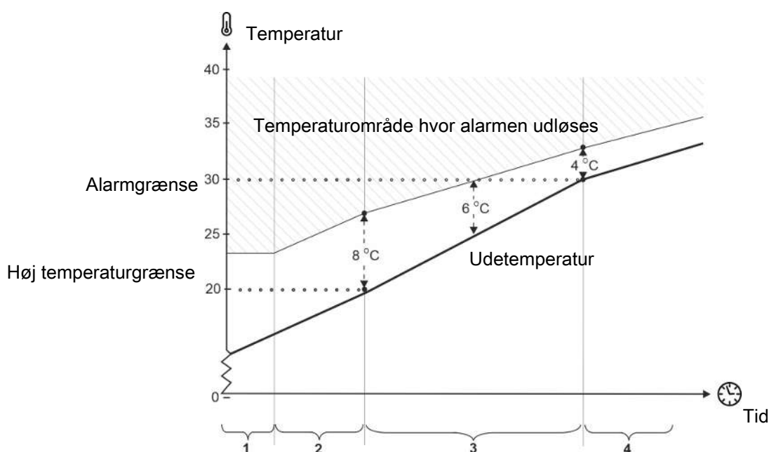
Figur 11: Sommertemperatur ved 20 °C og 30 °C ude
