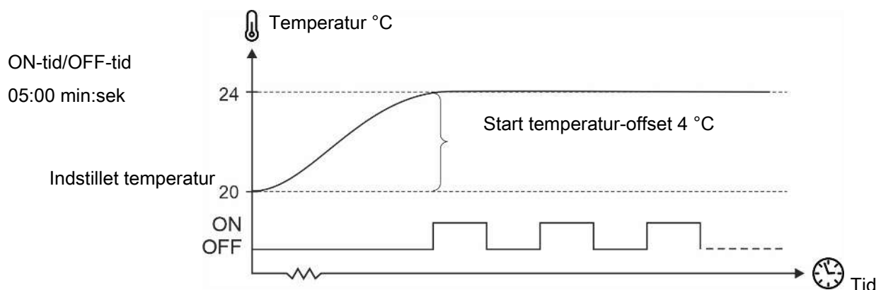
Figur 3: Relæstyret luftomrører (ON/OFF) styret efter temperatur
