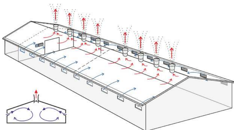
Рисунок 20: Поток воздуха в теории для боковой вентиляции.
