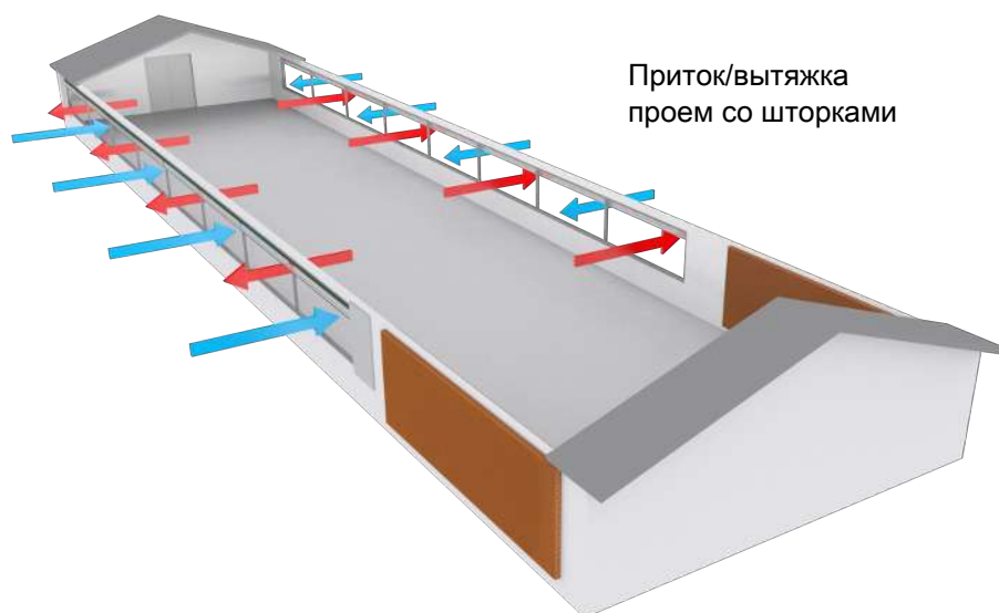
Рисунок 22: Пример помещения с естественной вентиляцией, применяемой вместе с туннельной вентиляцией, естественная вентиляция.
