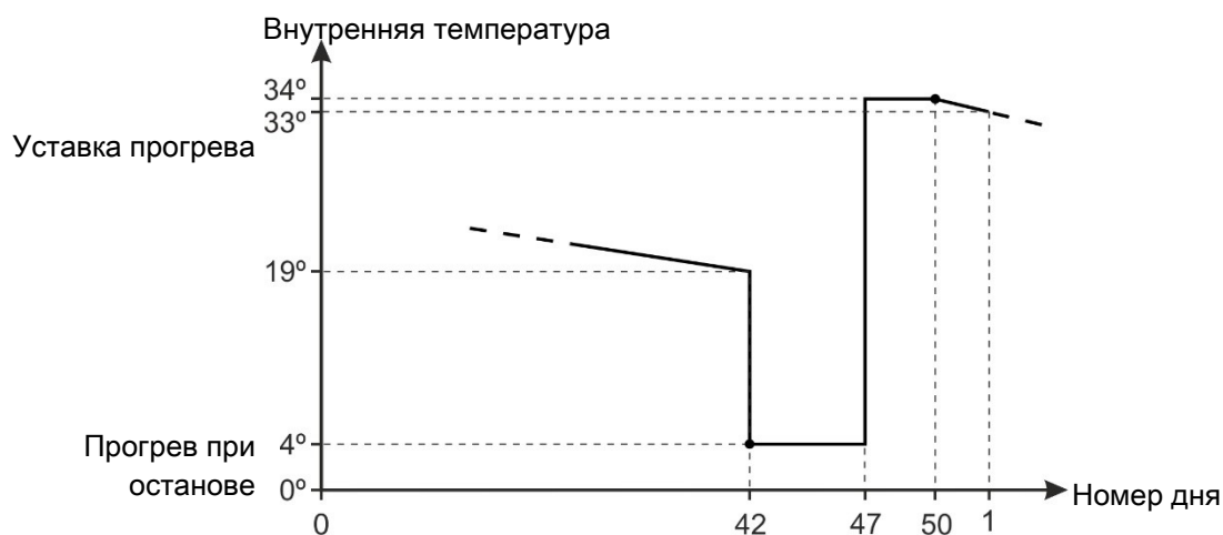
Рисунок 45: Пример настройки прогрева.
