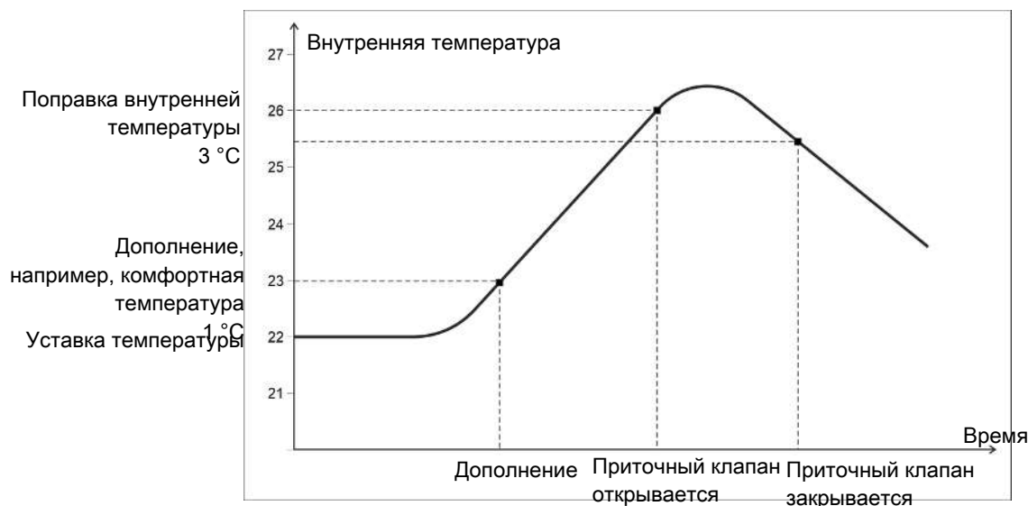
Рисунок 6: Комбидиффузный приточный клапан – регулировка внутренней температуры
