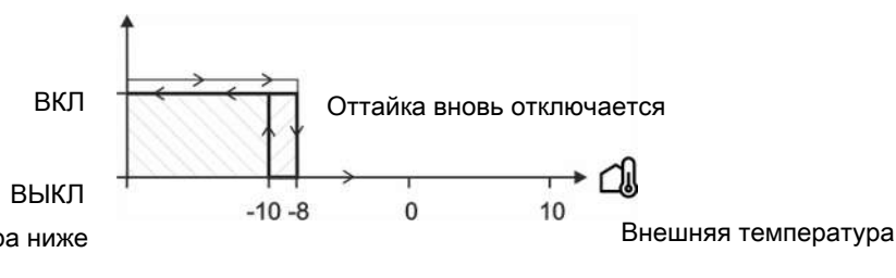
Рисунок 27: Активация оттайки
