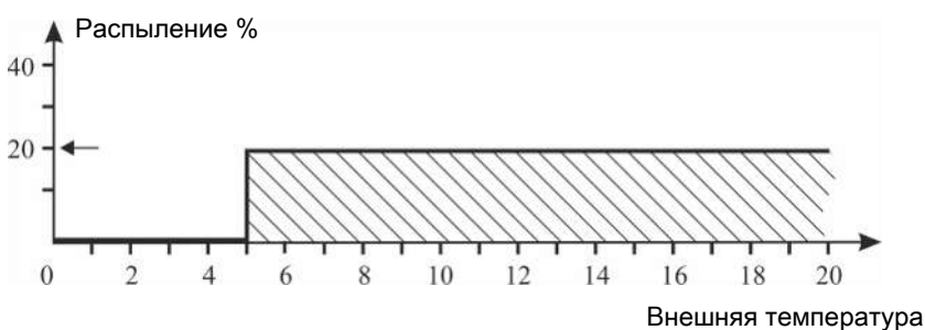
Рисунок 33: Распыление согласно внешней температуре
