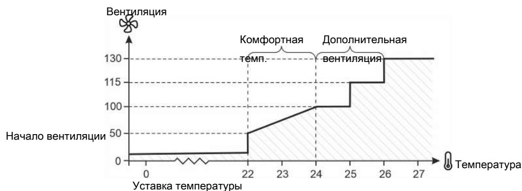
Рисунок 9: Дополнительная вентиляция активируется при превышении температуры внутри помещения выше значения, получаемого в результате сложения значений Уставки температуры и Комфортной температуры, а вентиляция уже работает на максимальном уровне. Контроллер условий микроклимата постепенно, ступенчато увеличивает дополнительную вентиляцию.
