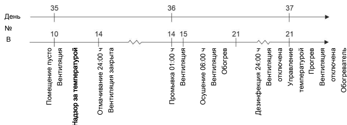
Рисунок 44: Последовательность промежуточных функций
