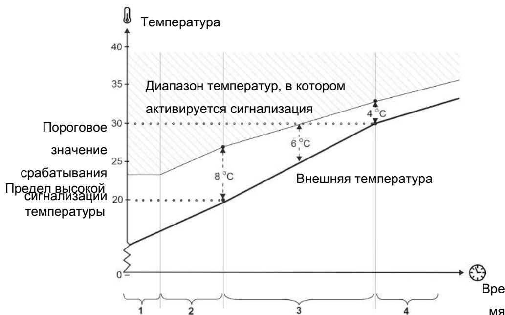
Рисунок 47: Летняя температура при 20° C и 30° C, снаружи
