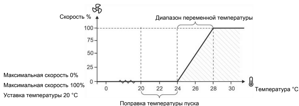
Рисунок 38: Подмешивающий вентилятор с управлением 0-10 В и положительной поправкой на температуру запуска.
