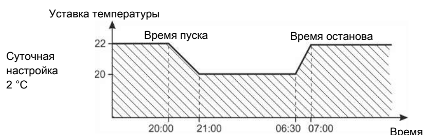
Рисунок 13: Дневная и ночная регулировка
