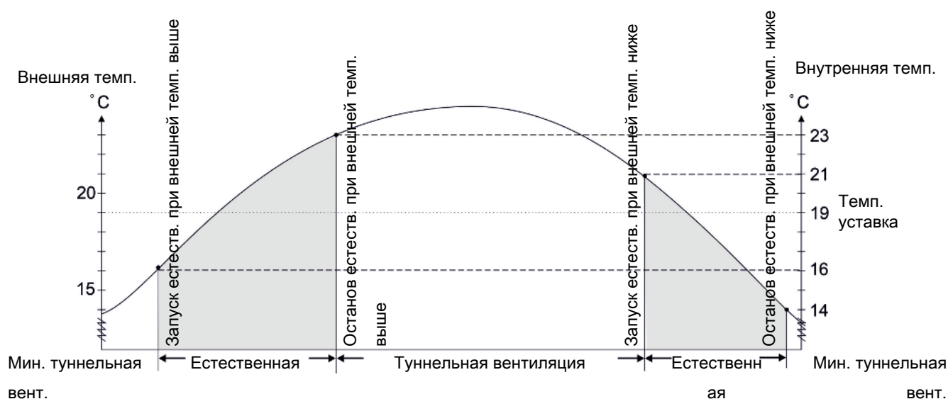
Рисунок 24: Естественная вентиляция активна в зависимости от текущей внешней температуры. Уставка температуры составляет 19 °C.
