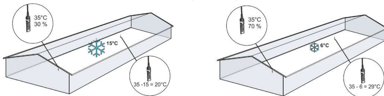
Рисунок 31: Чем ниже внешняя влажность, тем выше потенциал охлаждения.
