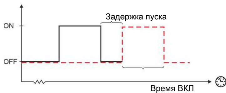
Рисунок 40: Контроль с помощью обогревателя
