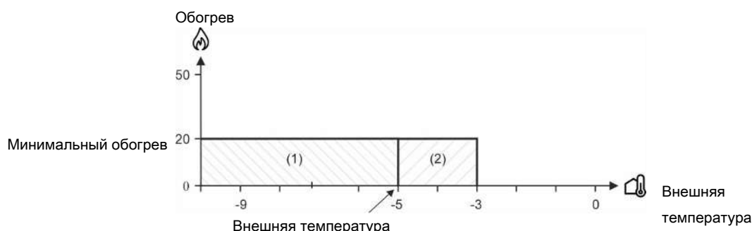
Рисунок 3: Минимальный обогрев при снижении или повышении температуры наружного воздуха
