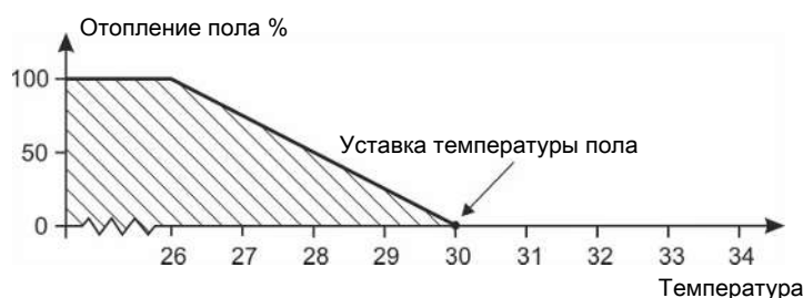
Рисунок 4: Обогрев пола с датчиком температуры
