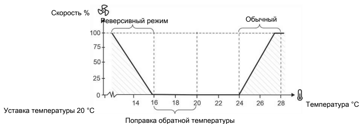
Рисунок 39: Управляемый с помощью 0–10 В подмешивающий вентилятор с реверсивным реле
