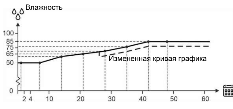
Рисунок 42: График влажности воздуха
