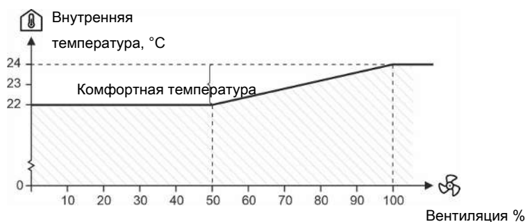
Рисунок 10: Комфортная температура при непрерывном производстве
