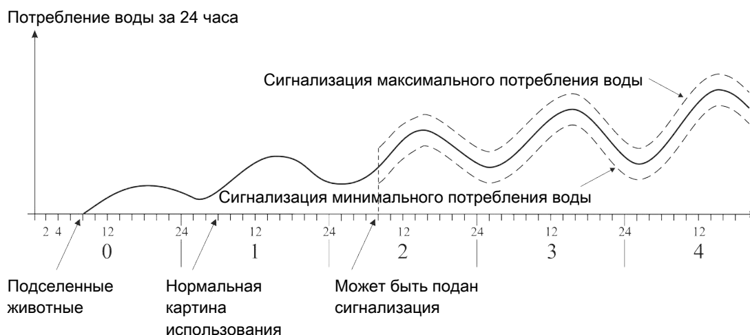
Рисунок 48: Пример сигнализации минимального и максимального потребления воды
