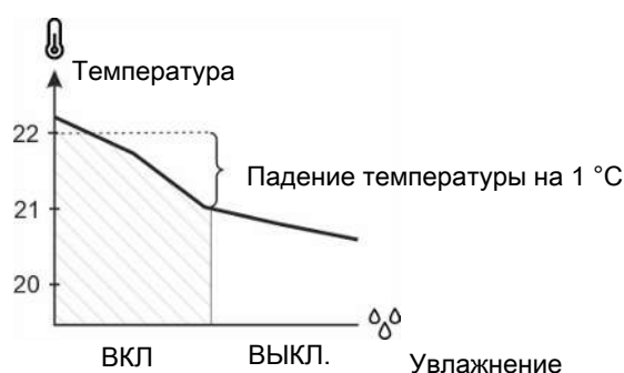
Рисунок 15: Понижение температуры: Увлажнение будет отключено, когда внутренняя температура будет на 1°C ниже уставки температуры. В противном случае увлажнение может вызвать дальнейшее снижение внутренней температуры.
