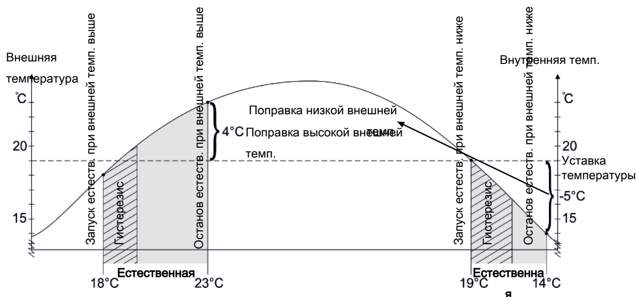
Рисунок 25: Естественная вентиляция активна в зависимости от текущей внешней температуры.
