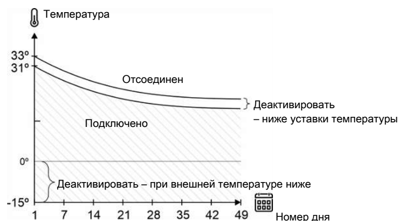
Рисунок 19: Рекуператор тепла – нижний и верхний пределы внешней температуры
