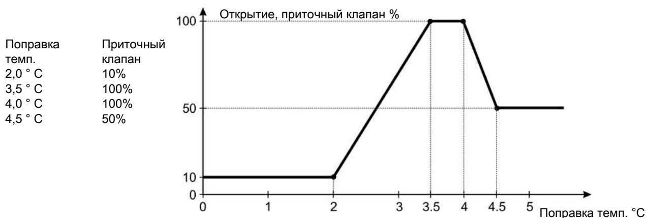
Рисунок 7: Комбидиффузный приточный клапан – уменьшение бесступенчатого открытия при высокой внешней температуре
