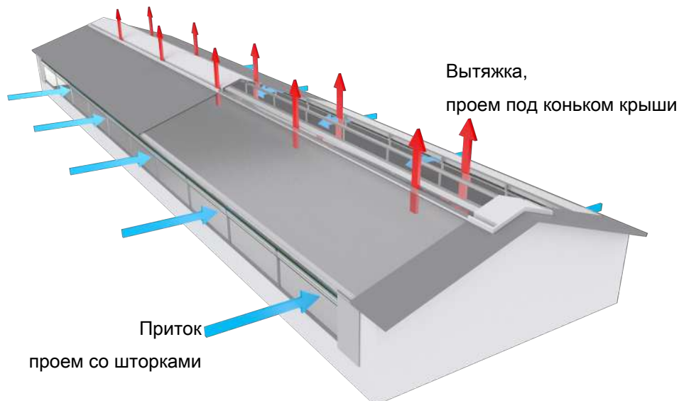
Рисунок 21: Например, в помещении, в котором используется только естественная вентиляция с проемами со шторками по бокам помещения и проемами под коньком крыши.
