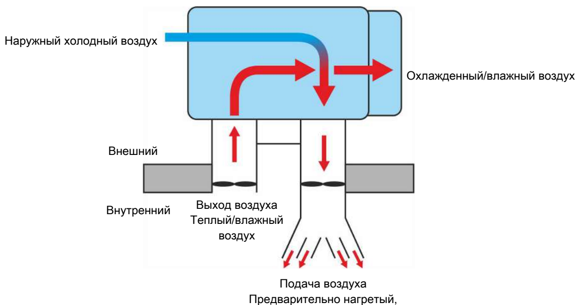
Рисунок 18: Пример работы принципа рекуператора тепла.
