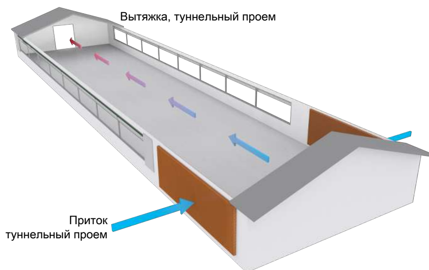
Рисунок 23: Пример помещения с естественной вентиляцией, применяемой вместе с туннельной вентиляцией, туннельная вентиляция.
