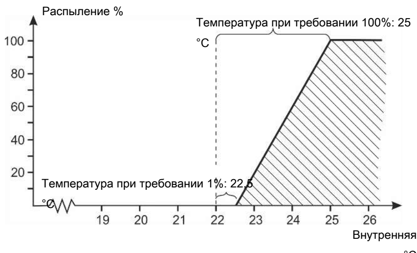
Рисунок 32: Распыление, в соответствии с внутренней температурой
