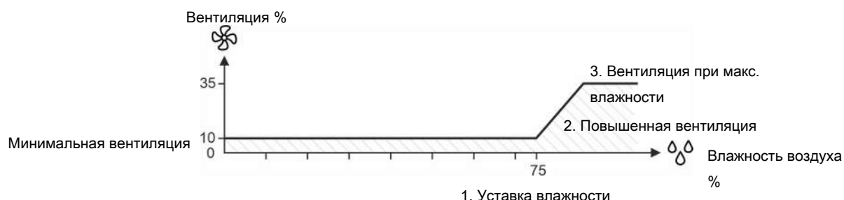
Рисунок 16: Вентиляция с увлажнением: 1. Влажность воздуха превышает уставку увлажнения 2. Контроллер помещения увеличивает вентиляцию. 3. Увеличьте вентиляцию до максимальной влажности (35%).
