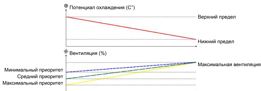
Рисунок 30: Чем выше потенциал охлаждения, тем выше приоритет раннего запуска охлаждения.
