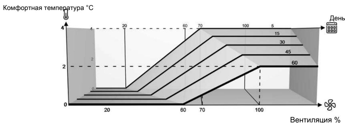
Рисунок 11: Комфортная температура при производстве партии
