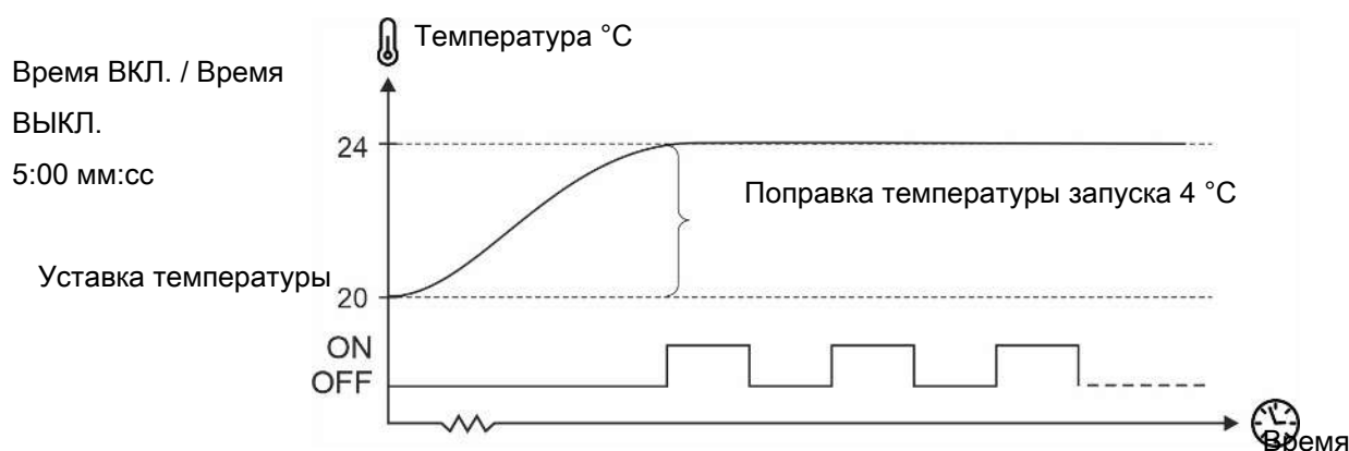
Рисунок 37: Подмешивающий вентилятор с релейным управлением (ВКЛ/ВЫКЛ), управляемый температурой
