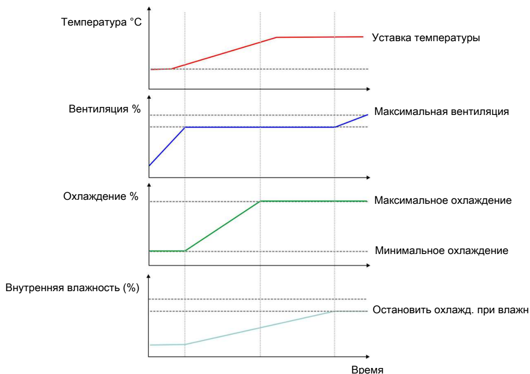
Рисунок 29: С целью поддержания требуемой внутренней температуры, охлаждение запускается до достижения уровнем вентиляции Максимальной вентиляции. Если охлаждение больше не сможет поддерживать температуру, вентиляция вновь увеличивается.
