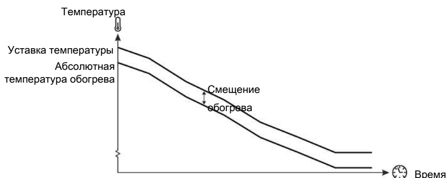
Рисунок 1: Настройка смещения обогрева
