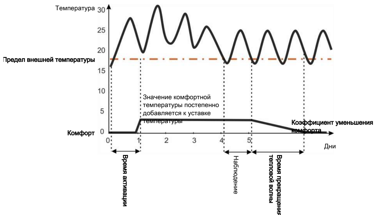
Рисунок 12: Комфортное значение тепловой волны
