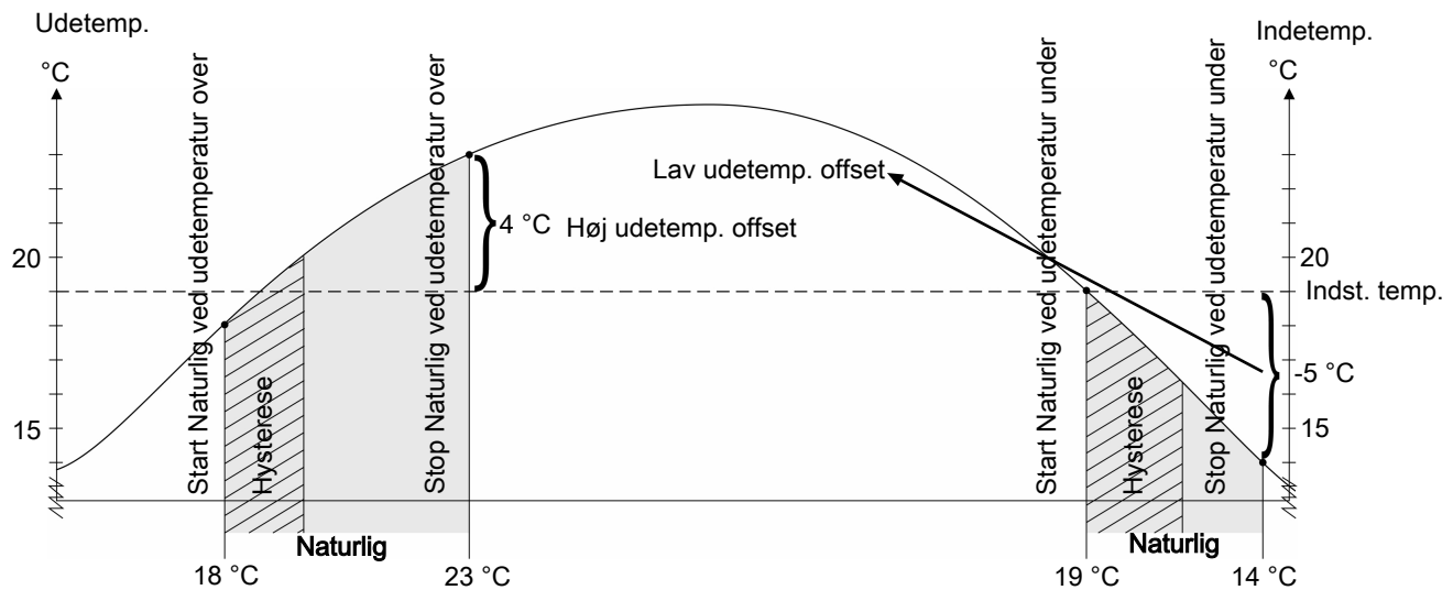
Figur 22: Naturlig ventilation er aktiv afhængig af den aktuelle udetemperatur.
