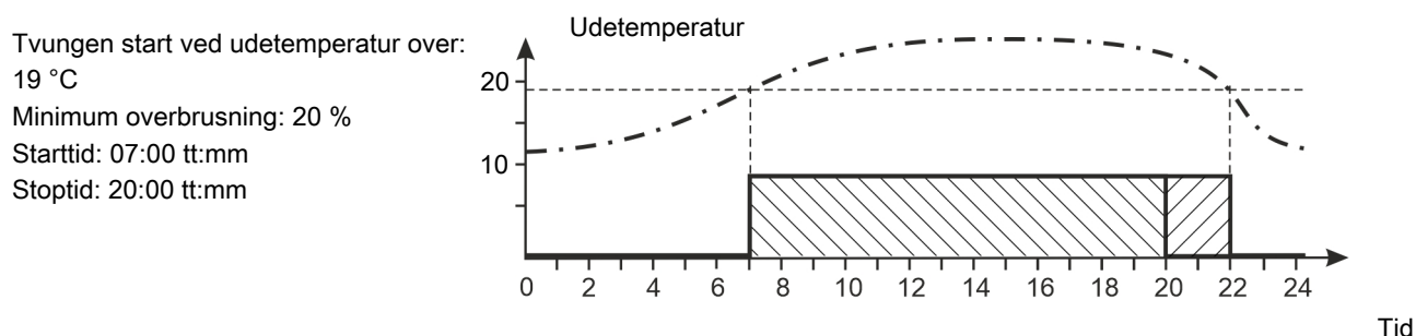
Figur 32: Overbrusning efter klokkeslæt og udetemperatur
