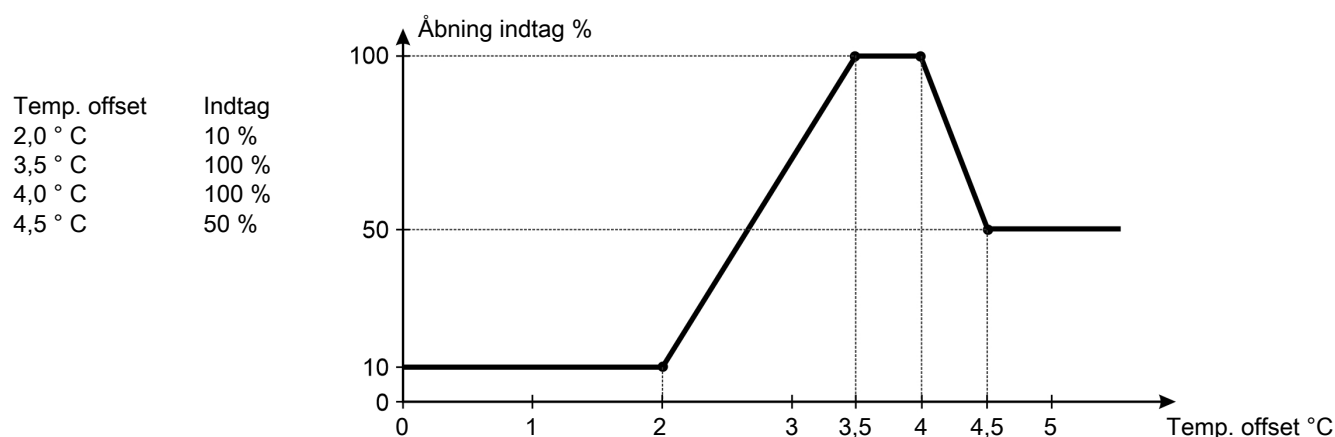
Figur 9: Combi-Diffus indtag – reduceret trinløs åbning ved høj udetemperatur
