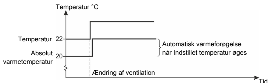
Figur 34: Varmetilsætning
