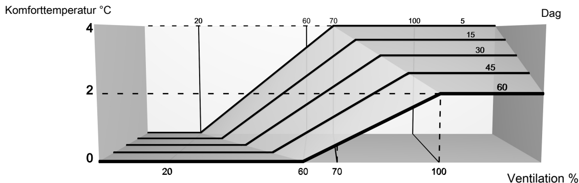
Figur 5: Komforttemperatur ved holddrift
