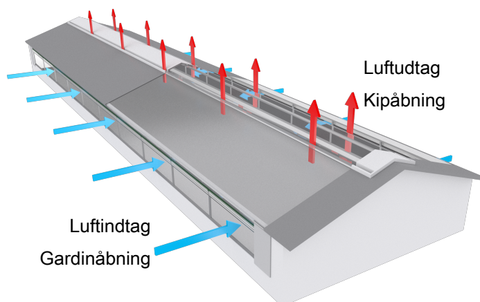
Figur 18: Eksempel på hus med ren Naturlig ventilation med gardinåbninger på husets sider og kipåbning i taget.
