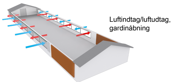
Figur 19: Eksempel på hus med Naturlig ventilation i kombination med tunnel ventilation, Naturlig ventilation.
