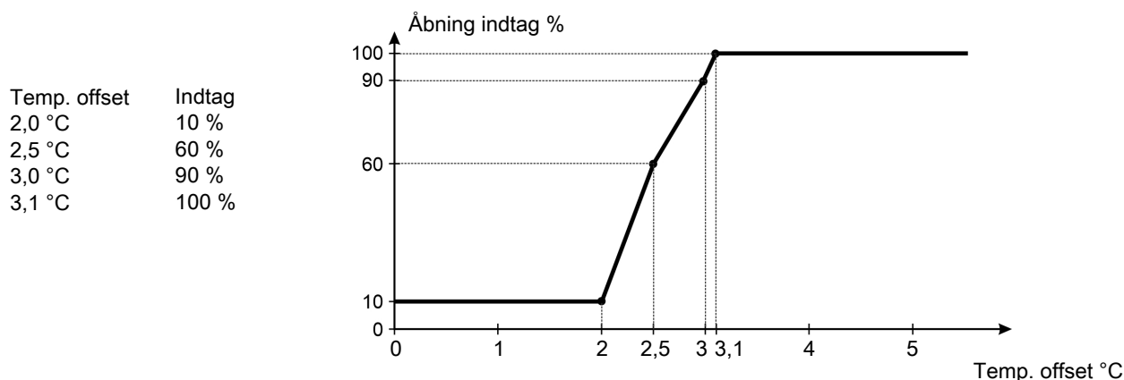
Figur 10: Combi-Diffus indtag – trinløs åbning ud fra inde- og udetemperatur
