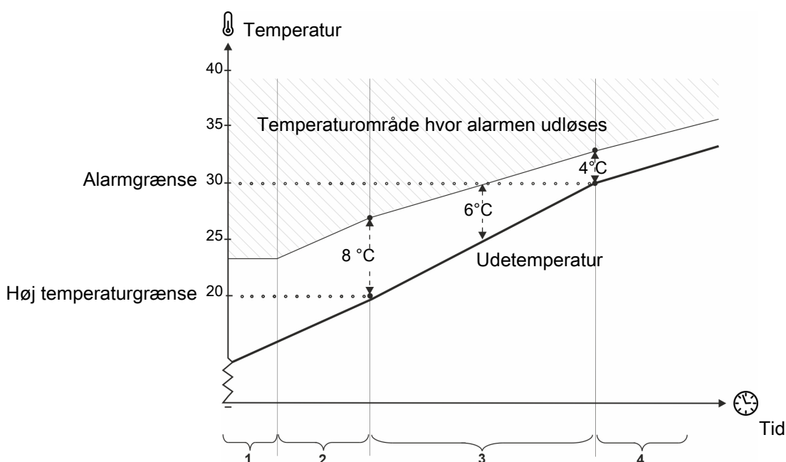
Figur 42: Sommertemperatur ved 20 °C og 30 °C ude
