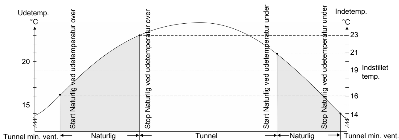
Figur 21: Naturlig ventilation er aktiv afhængig af den aktuelle udetemperatur. Indstillet temperatur 19 °C.
