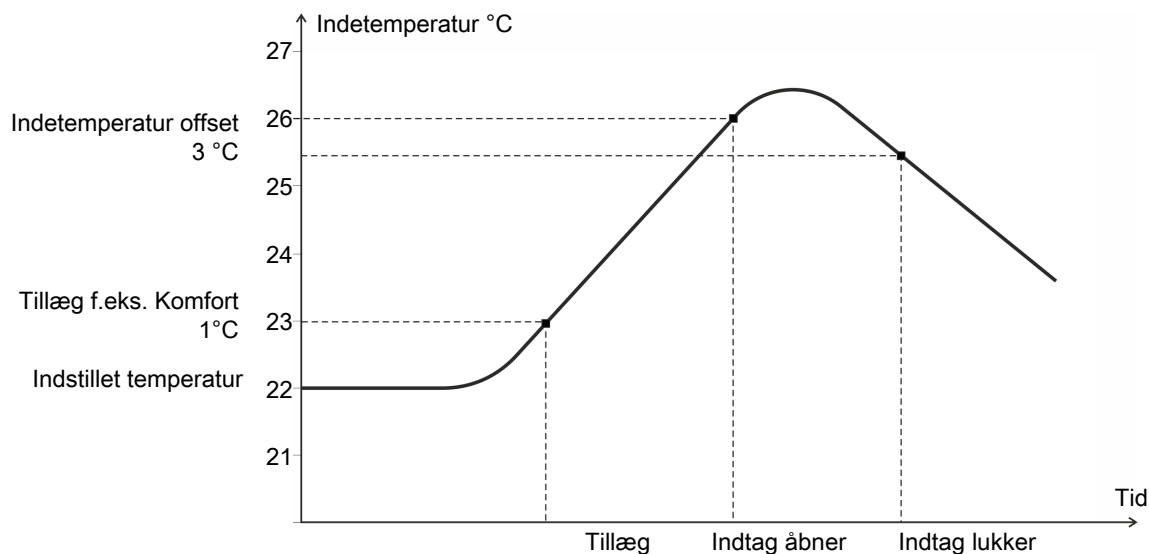
Figur 8: Combi-diffus indtag – indetemperatur-reguleret
