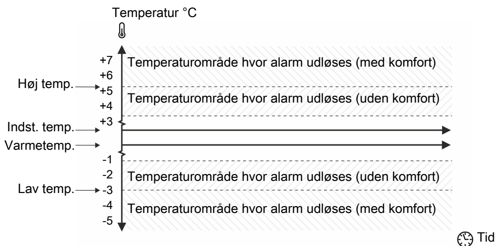
Figur 41: Alarm høj og lav temperatur
