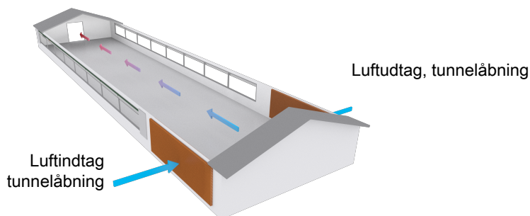
Figur 20: Eksempel på hus med Naturlig ventilation i kombination med tunnel ventilation, Tunnelventilation.
