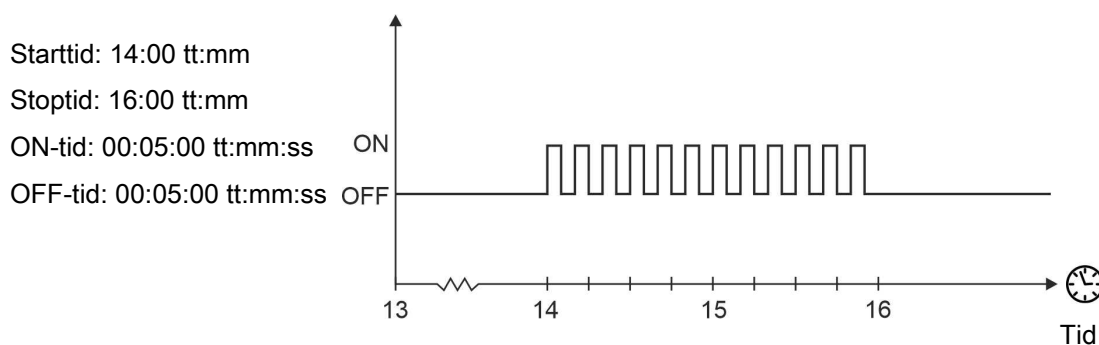
Figur 24: Døgnursregulering
