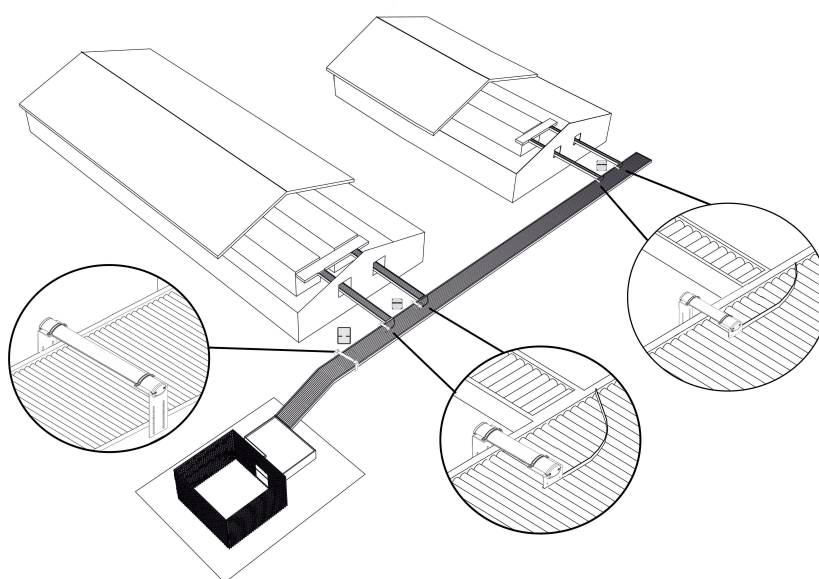
Figure 16: Schéma pour le placement des compteurs d'œufs automatiques.
