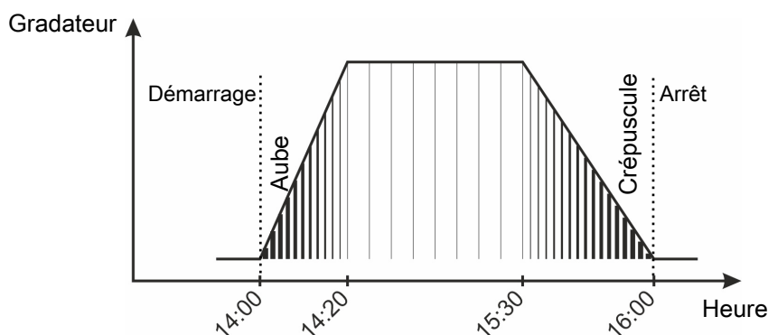
Figure 11: Gradateur normal d'éclairage Aube et crépuscule sont intégrés dans la période d'éclairage.
