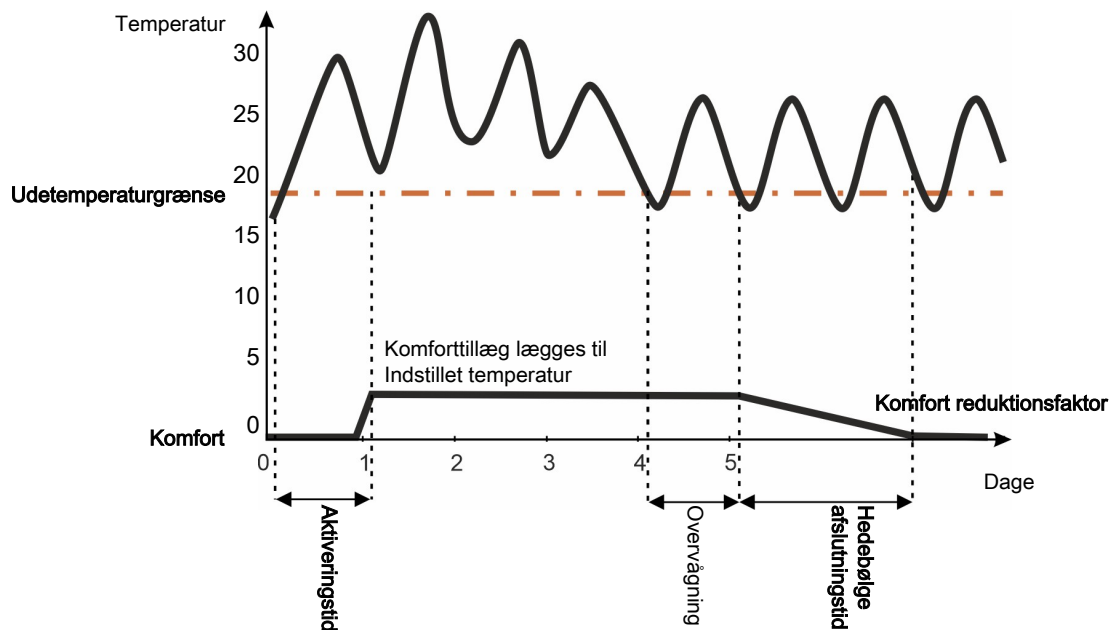
Figur 5: Hedebølge-komfort
