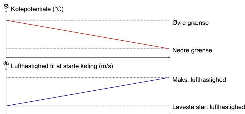
Figur 32: I områder med lav udefugt og et stort kølepotentiale, kan kølingen starte ved en lavere lufthastighed. Omvendt vil man i områder med lavt kølepotentiale vente så længe som muligt med at starte kølingen, så den starter ved maksimum lufthastighed.
