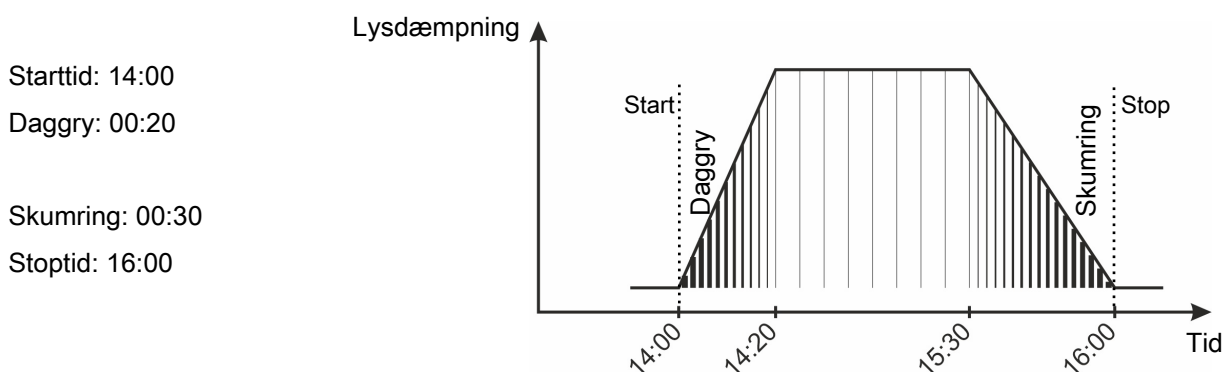
Figur 40: Normal lysdæmpning. Daggry og skumring ligger inde i lys-perioden.
