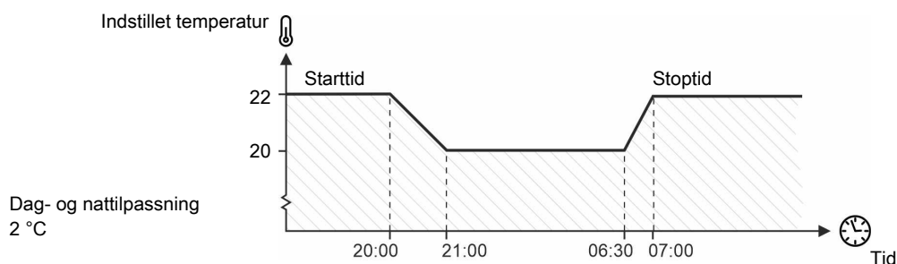
Figur 8: Dag- og nattilpasning indstillet som en natlig temperatursænkning.
