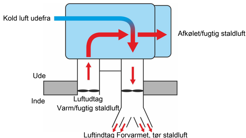
Figur 14: Eksempel på varmegenvinder-princip.
