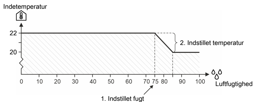
Figur 12: Fugtstyring med temperatursænkning
