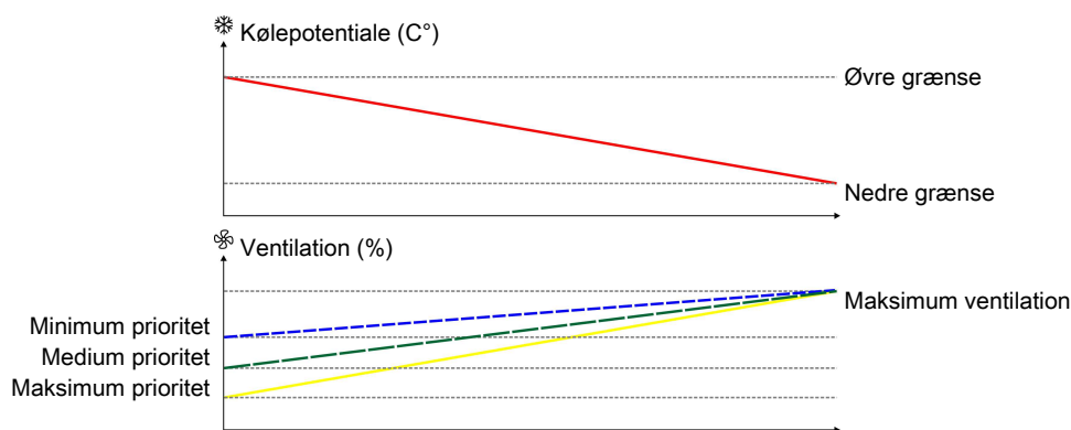
Figur 27: Jo højere kølepotentiale, desto højere prioritet på tidlig start af køling.
