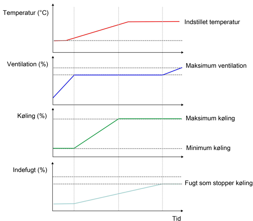
Figur 26: For at holde den ønskede indetemperatur starter kølingen allerede, inden ventilationsniveauet når Maksimum ventilation. Når kølingen ikke kan holde temperaturen, øges ventilationen igen.
