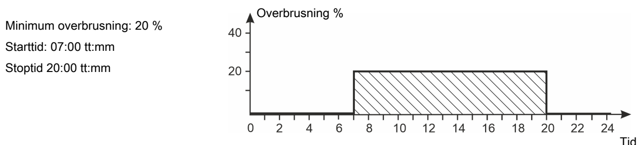
Figur 30: Overbrusning efter klokkeslæt
