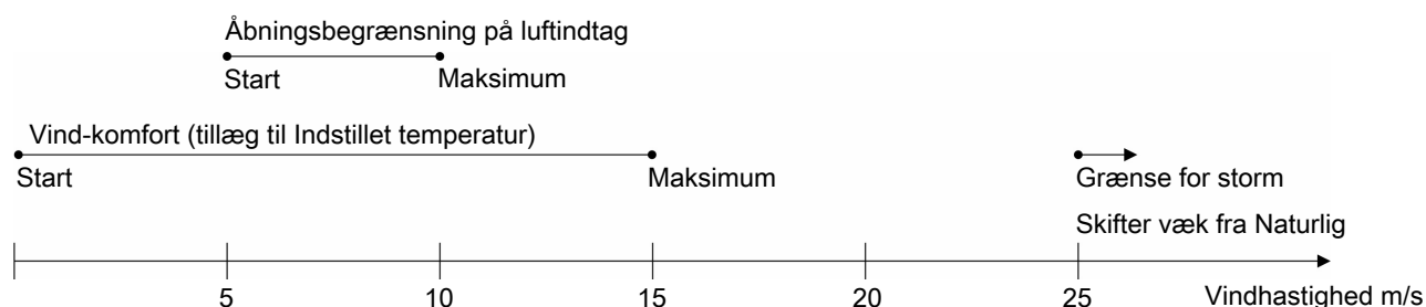
Figur 22: Naturlig ventilation ved stigende vindhastigheder
