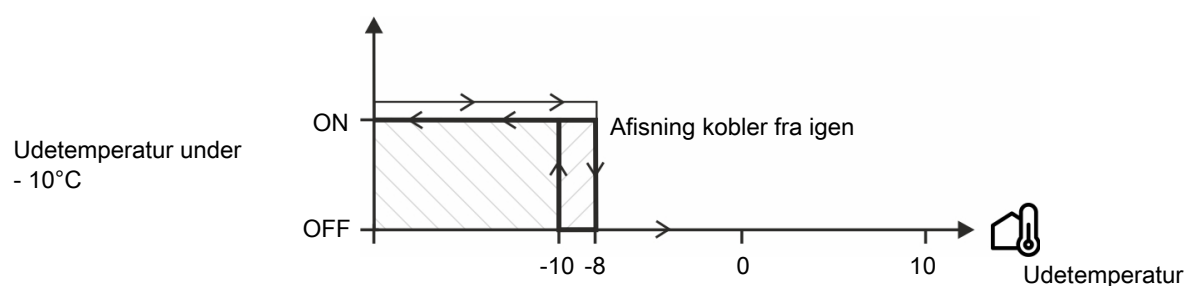
Figur 13: Aktivering af afisning
