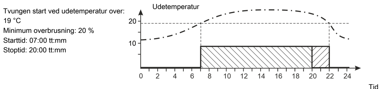
Figur 31: Overbrusning efter klokkeslæt og udetemperatur
