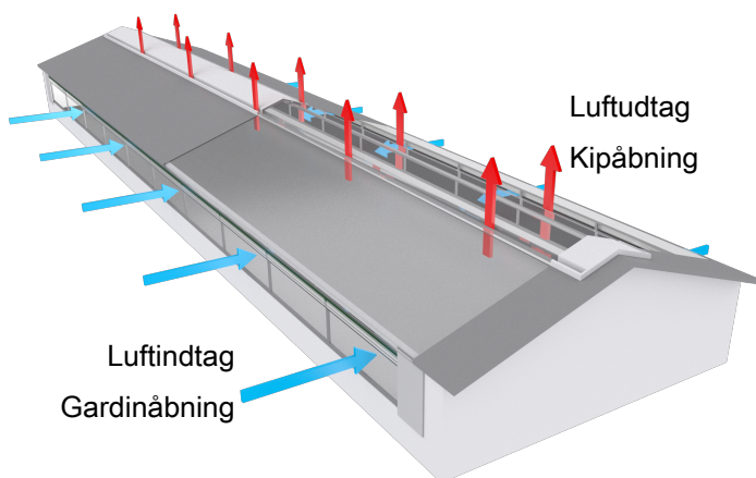
Figur 17: Eksempel på hus med ren Naturlig ventilation med gardinåbninger på husets sider og kipåbning i taget.
