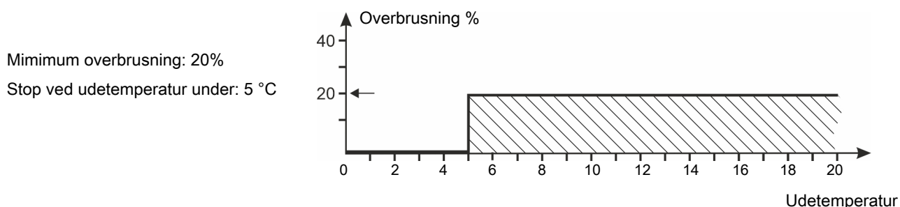
Figur 29: Overbrusning efter udetemperatur
