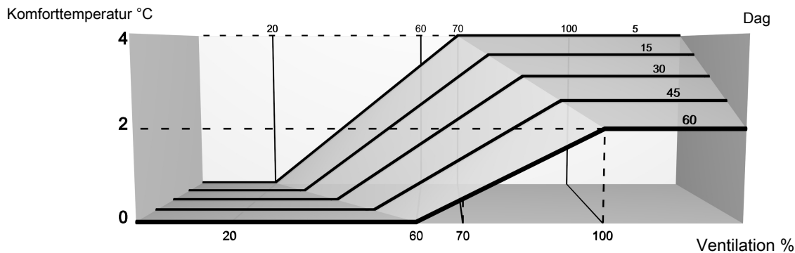
Figur 6: Komforttemperatur ved holddrift
