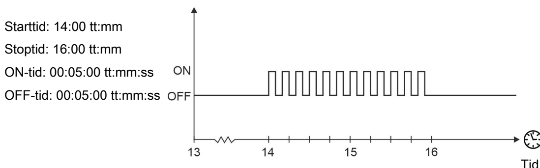
Figur 23: Døgnursregulering
