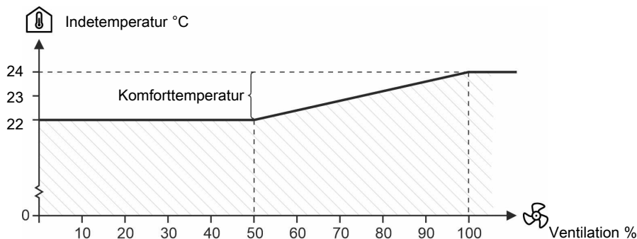
Figur 7: Komforttemperatur ved kontinuerlig drift
