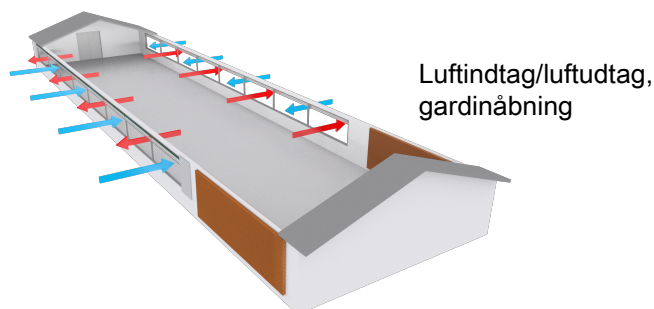
Figur 18: Eksempel på hus med Naturlig ventilation i kombination med tunnel ventilation, Naturlig ventilation.
