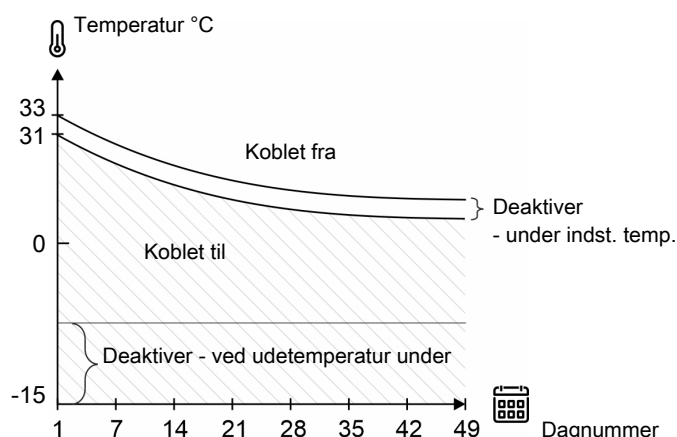
Figur 15: Varmegenvinder – lav og høj udetemperaturgrænse
