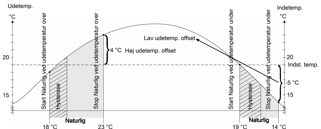
Figur 21: Naturlig ventilation er aktiv afhængig af den aktuelle udetemperatur.
