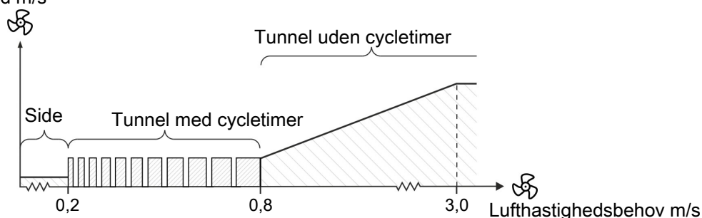
Figur 16: Ventilationsforløb med cycletimer ved tunnel-ventilation
