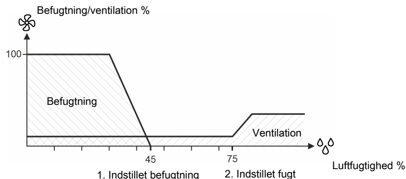
Figur 9: 1. Faldende luftfugtighed. Luftfugtigheden er under Indstillet befugtning. Staldcomputeren starter befugtningen. 2. Stigende luftfugtighed. Luftfugtigheden er over Indstillet fugt. Staldcomputeren øger ventilationen.
