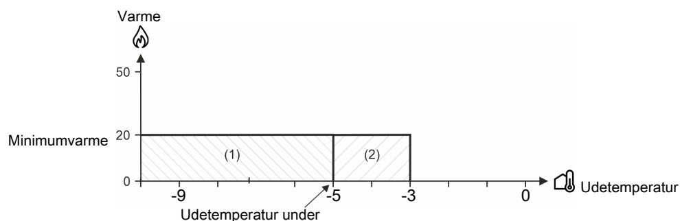
Figur 36: Minimumvarme ved faldende eller stigende udetemperatur
