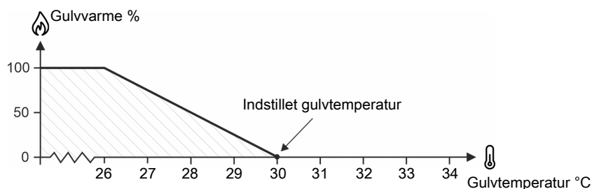
Figur 37: Gulvvarme med temperaturføler
