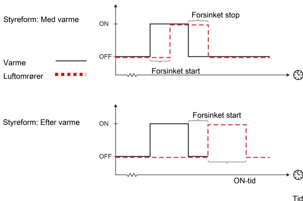
Figur 24: Varmekilderegulering
