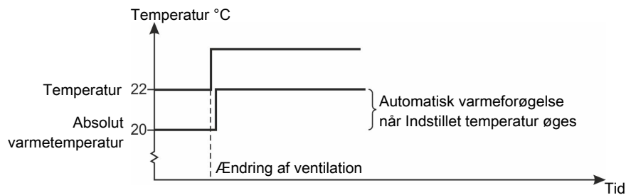
Figur 35: Varmetilsætning
