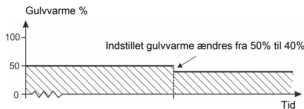
Figur 38: Gulvvarme uden temperaturføler
