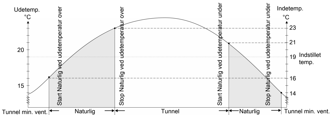
Figur 20: Naturlig ventilation er aktiv afhængig af den aktuelle udetemperatur. Indstillet temperatur 19 °C.
