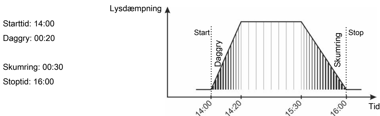
Figur 13: Normal lysdæmpning. Daggy og skumring ligger inde i lys-perioden.
