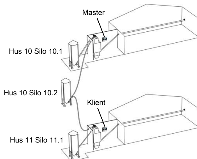
Figur 16: Eksempel på silo delt mellem to huse med staldcomputere på LAN-netværk.
