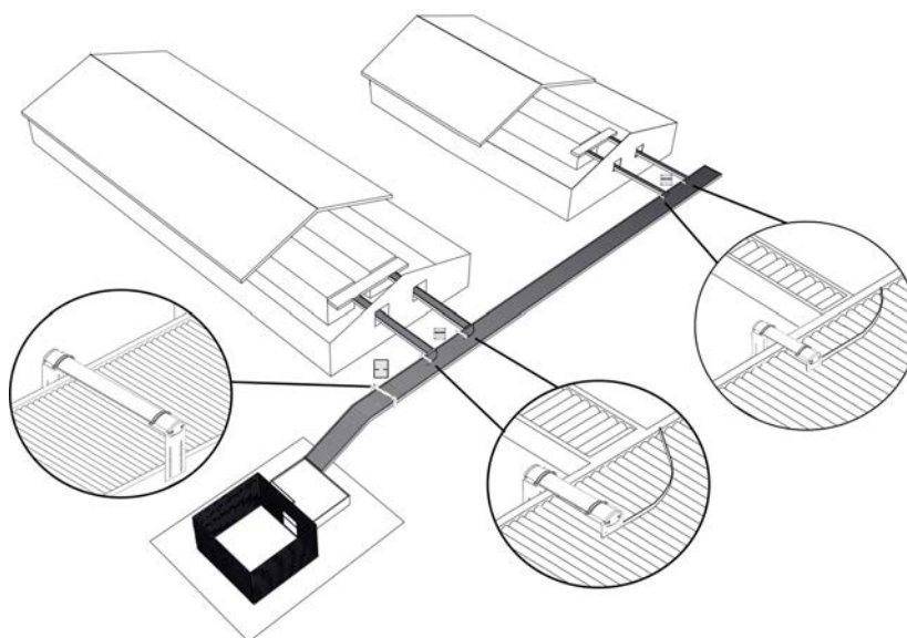
Figur 18: Principtegning for placering af automatiske ægtællere.
