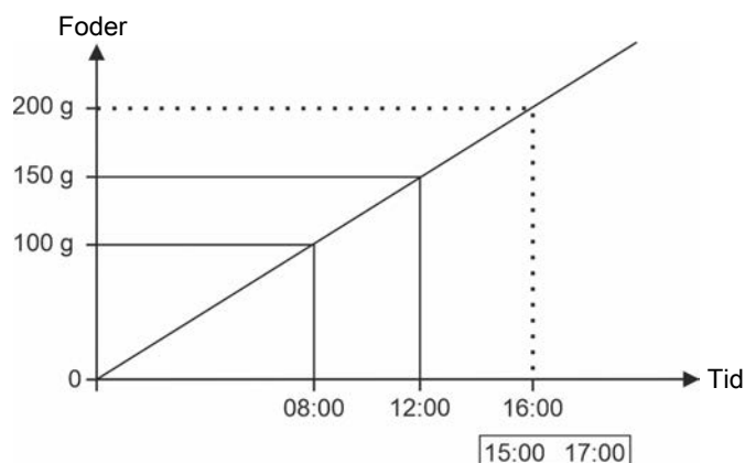
Figur 8: Den sidste fodring starter indenfor den indstillede adaptive foderperiode.
