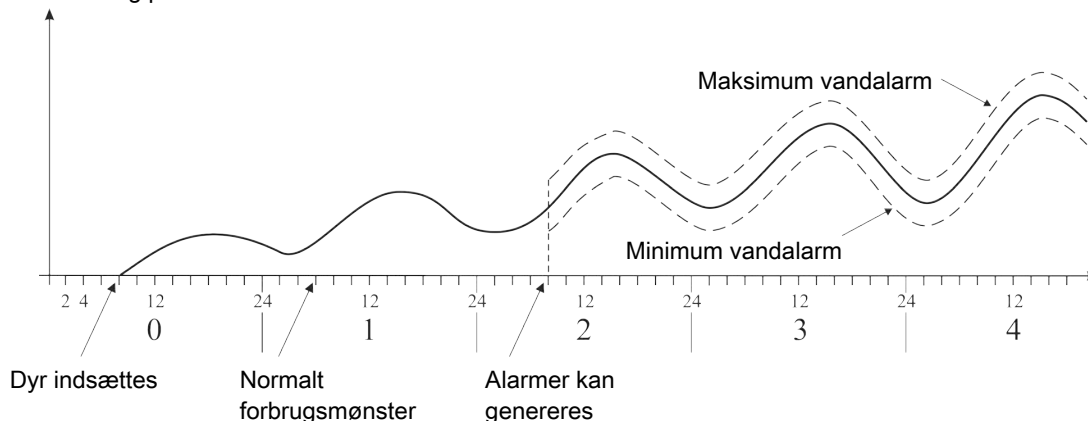
Figur 19: Eksempel på minimum og maksimum vandalarm
