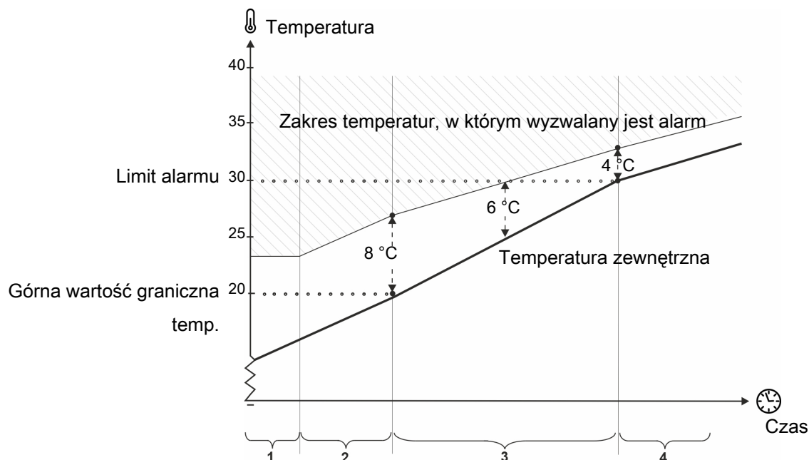
Rysunek 42: Temperatura letnia przy 20°C i 30°C na zewnątrz
