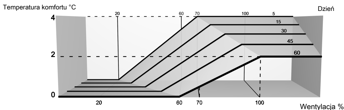
Rysunek 5: Temperatura komfortu przy produkcji tuczu
