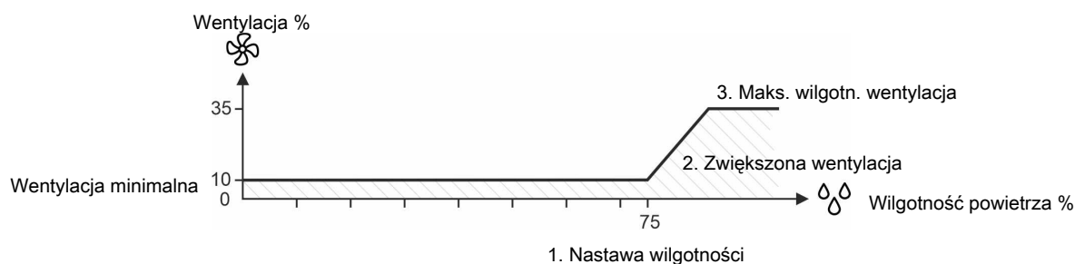
Rysunek 13: Regulowanie wilgotności przez wentylację: 1. Wilgotność powietrza przekracza nastawę wilgotności. 2. Sterownik zwiększa wentylację. 3. Zwiększenie wentylacji do regulowania wilgotności do wartości maksymalnej (35%).
