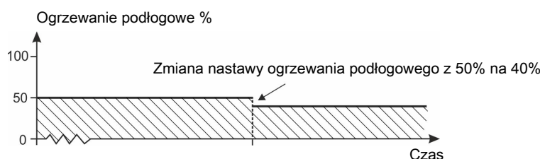
Rysunek 37: Ogrzewanie podłogowe bez czujnika temperatury
