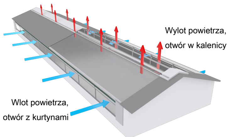
Rysunek 18: Przykładowo w budynku z czystą wentylacją naturalną z otworami z kurtynami po obu stronach i otworu w kalenicy.
