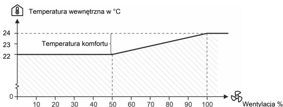
Rysunek 6: Temperatura komfortu przy produkcji ciągłej
