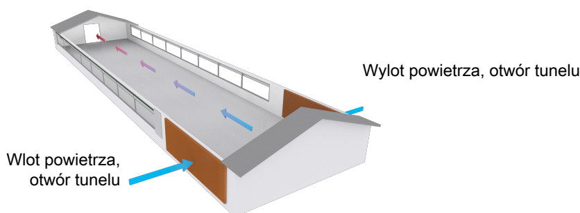
Rysunek 20: Przykład budynku inwentarskiego z wentylacją naturalną w połączeniu z wentylacją tunelową — wentylacja tunelowa.
