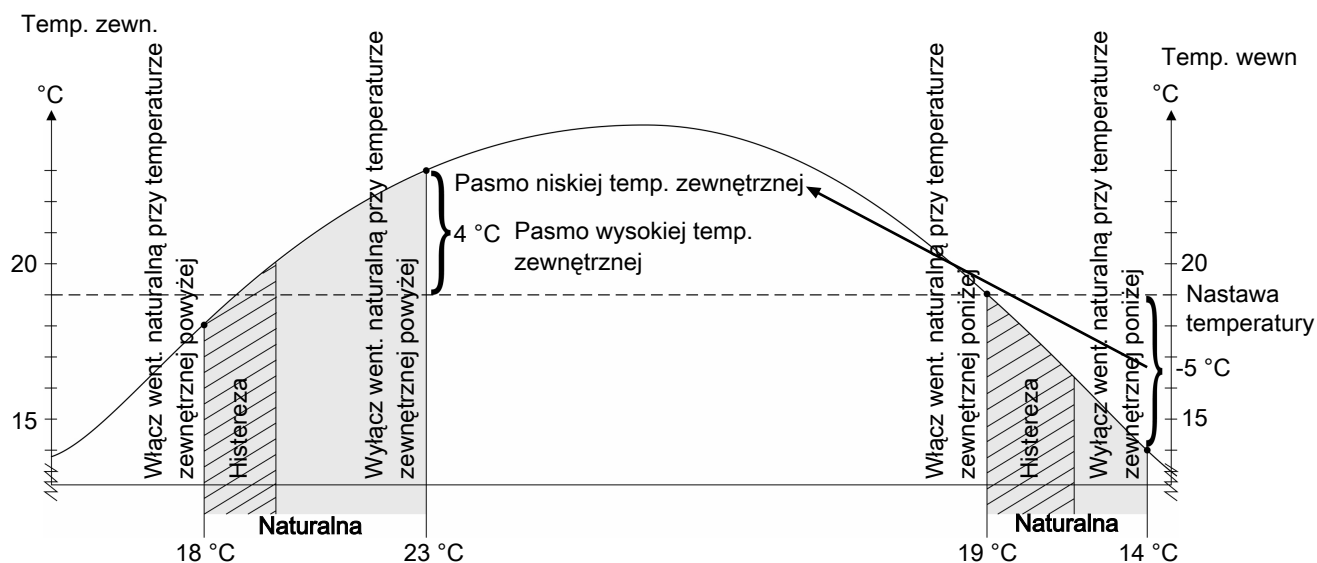
Rysunek 22: Wentylacja naturalna jest aktywna w zależności od aktualnej temperatury zewnętrznej.
