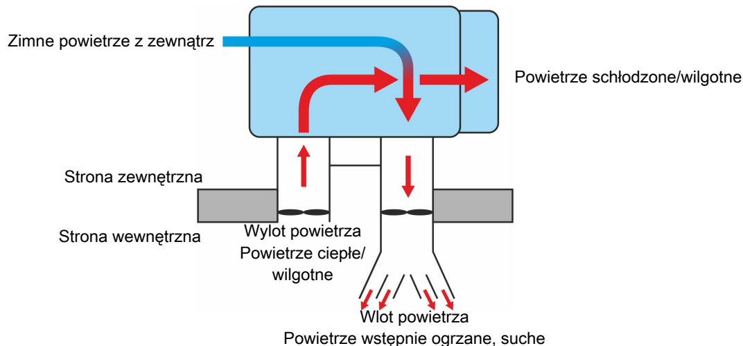
Rysunek 16: Przykład zasady działania centrali wentylacyjnej.
