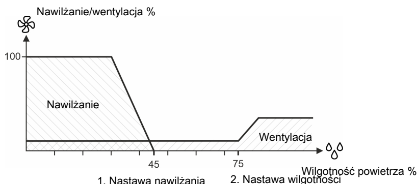
Rysunek 11: 1. Zmniejszenie wilgotności powietrza. Wilgotność powietrza jest niższa od wartości nastawy nawilżania. Sterownik rozpoczyna nawilżanie. 2. Zwiększenie wilgotności powietrza. Wilgotność powietrza jest wyższa od wartości nastawy wilgotności. Sterownik zwiększa wentylację.
