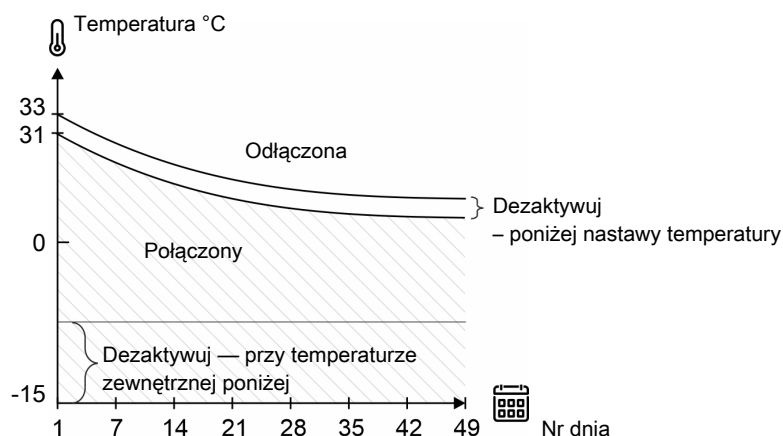
Rysunek 17: Centrala wentylacyjna – dolne i górne wartości graniczne temp. zewnętrznej
