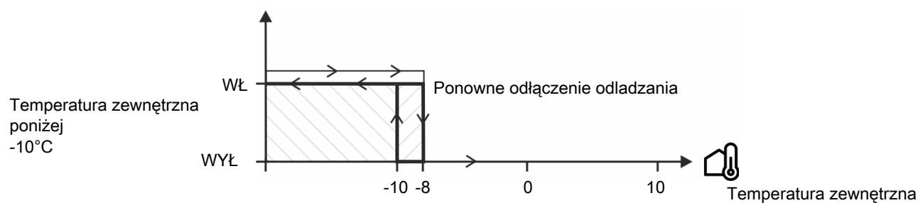
Rysunek 15: Aktywacja funkcji odmrażania
