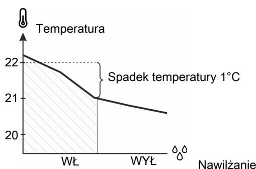
Rysunek 12: Obniżenie temperatury: Nawilżanie zostanie dezaktywowane, jeśli temperatura wewnętrzna wynosi 1°C poniżej wartości Nastawy temperatury. W przeciwnym razie nawilżanie mogłoby spowodować dalszy spadek temperatury wewnętrznej.
