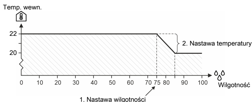
Rysunek 14: Sterowanie wilgotnością poprzez obniżenie temperatury
