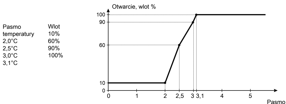
Rysunek 10: Wlot wentylacji łączonej — bezstopniowe otwieranie w zależności od temperatury wewnętrznej i zewnętrznej Wlot otwiera się, gdy temperatura wewnętrzna przekroczy Nastawę temperatury + dowolne dodatki, przykładowo Temperaturę komfortu o liczbę stopni, do jakiej ustawiona jest wartość Pasma temperatury wewnętrznej oraz gdy temperatura zewnętrzna jest powyżej limitu Temperatury zewnętrznej .
