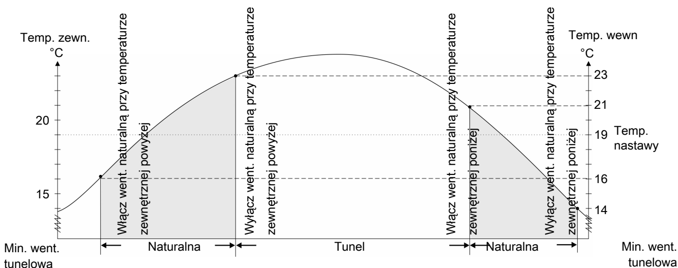
Rysunek 21: Wentylacja naturalna jest aktywna w zależności od aktualnej temperatury zewnętrznej. Nastawa temperatury wynosi 19°C.
