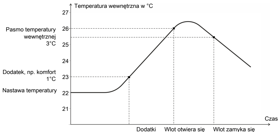
Rysunek 8: Wlot wentylacji łączonej — regulowana temperatura wewnętrzna
