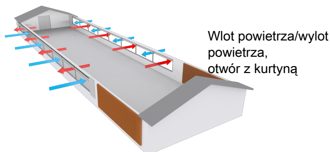
Rysunek 19: Przykład budynku inwentarskiego z wentylacją naturalną w połączeniu z wentylacją tunelową — wentylacja naturalna.
