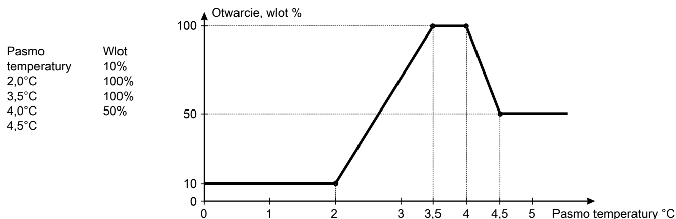
Rysunek 9: Wlot wentylacji łączonej — redukcja bezstopniowego otwierania przy wysokiej temperaturze zewnętrznej
