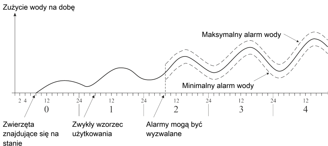
Rysunek 43: Przykład minimalnego i maksymalnego alarmu wody
