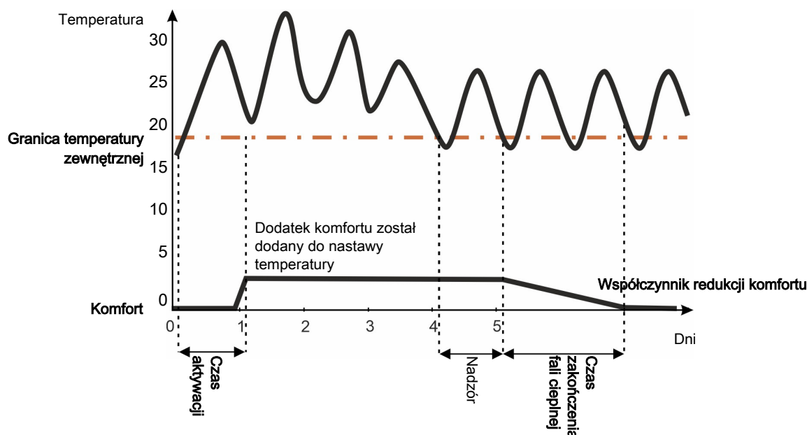
Rysunek 4: Komfort fali ciepłej
