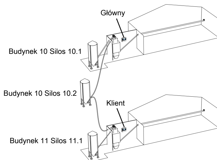
Rysunek 14: Przykład silosu współdzielonego między dwoma budynkami połączonymi ze sterownikami w sieci LAN.
