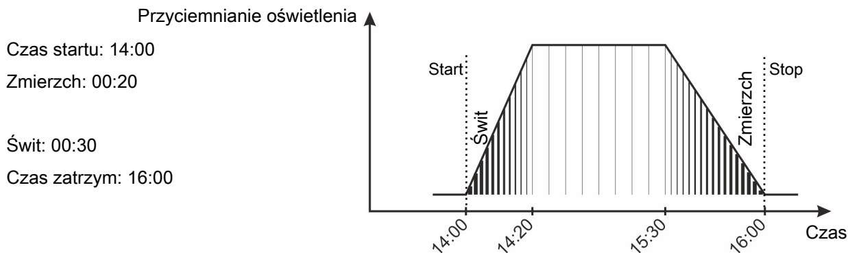
Rysunek 40: Funkcja normalnego przyciemniania oświetlenia Świt i zmierzch jest uwzględniona w cyklu oświetlenia.
