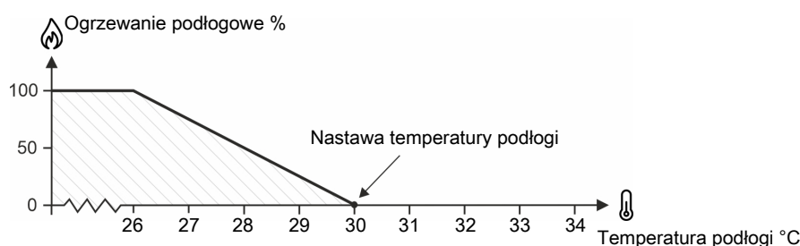
Rysunek 37: Ogrzewanie podłogowe z czujnikiem temperatury
