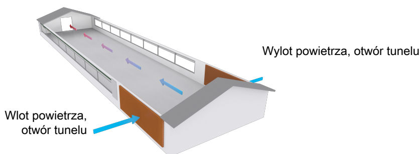
Rysunek 19: Przykład budynku inwentarskiego z wentylacją naturalną w połączeniu z wentylacją tunelową — wentylacja tunelowa.
