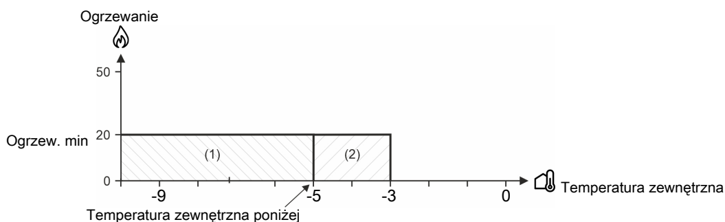
Rysunek 36: Minimalne ogrzewanie przy obniżającej się lub wzrastającej temperaturze zewnętrznej
