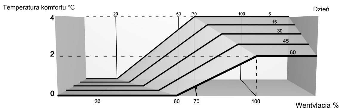
Rysunek 6: Temperatura komfortu przy produkcji tuczu
