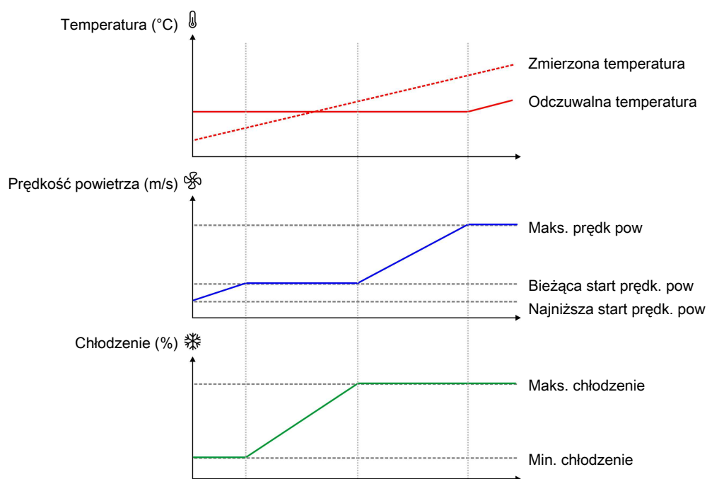
Rysunek 33: Chłodzenie rozpoczyna się już z niską prędkością powietrza, aby utrzymać żądaną temperaturę wewnętrzną. Jeśli chłodzenie nie może utrzymać temperatury, prędkość powietrza ponownie wzrasta.
