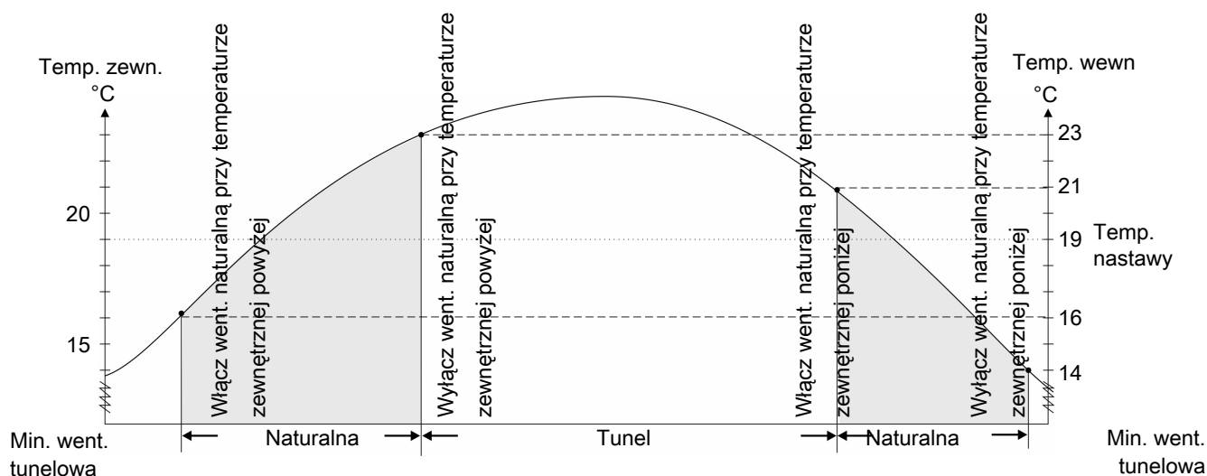
Rysunek 20: Wentylacja naturalna jest aktywna w zależności od aktualnej temperatury zewnętrznej. Nastawa temperatury wynosi 19°C.
