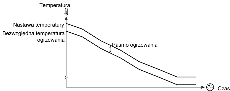
Rysunek 34: Ustaw pasmo ogrzewania
