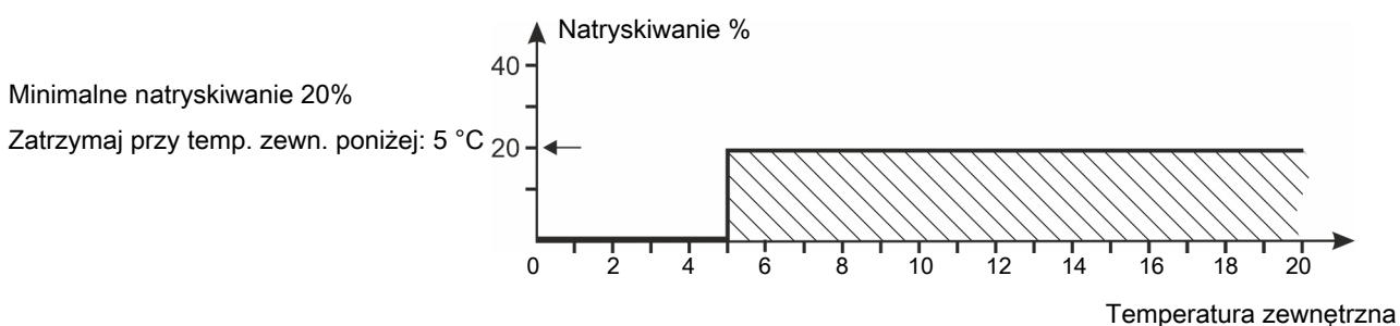
Rysunek 29: Natryskiwanie zgodnie z temperaturą zewnętrzną
