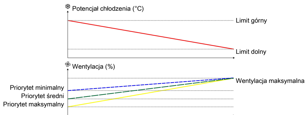
Rysunek 27: Im wyższy potencjał chłodzenia, tym wyższy priorytet wczesnego rozpoczęcia chłodzenia.
