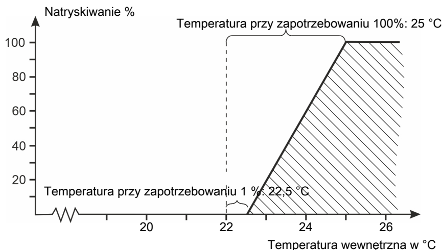
Rysunek 28: Natryskiwanie zgodnie z temperaturą wewnętrzną
