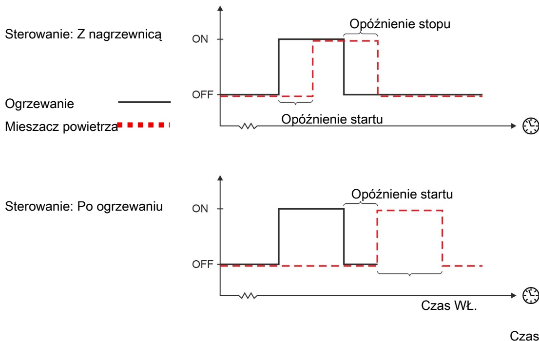
Rysunek 24: Sterownik z nagrzewnicą
