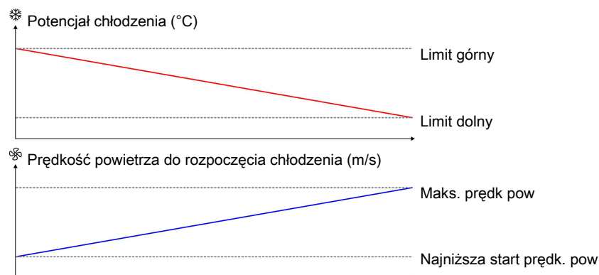
Rysunek 32: W obszarach o niskiej wilgotności zewnętrznej oraz dużym potencjale chłodzenia, chłodzenie może rozpocząć się przy niższych prędkościach powietrza. Natomiast w obszarach o niskim potencjale chłodzenia, chłodzenie rozpocznie się najpóźniej, jak to możliwe, co oznacza, że rozpoczyna się przy maksymalnej prędkości powietrza.
