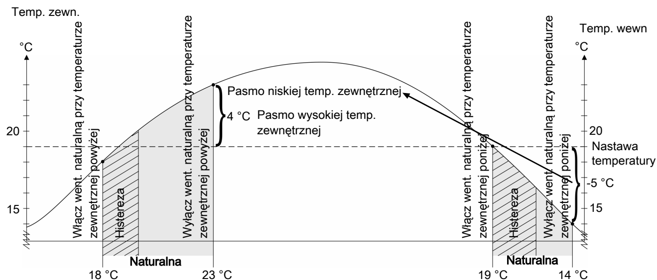
Rysunek 21: Wentylacja naturalna jest aktywna w zależności od aktualnej temperatury zewnętrznej.
