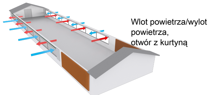
Rysunek 18: Przykład budynku inwentarskiego z wentylacją naturalną w połączeniu z wentylacją tunelową — wentylacja naturalna.
