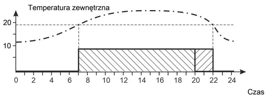
Rysunek 31: Natryskiwanie zgodnie z czasem i temperaturą zewnętrzną
