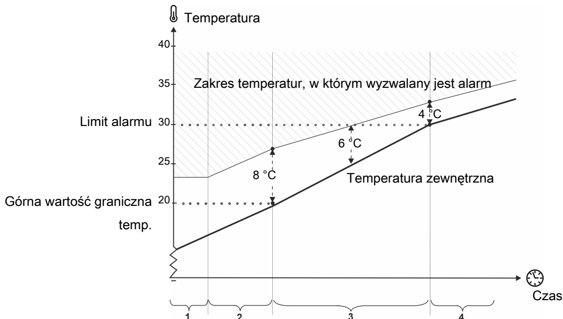
Rysunek 43: Temperatura letnia przy 20°C i 30°C na zewnątrz
