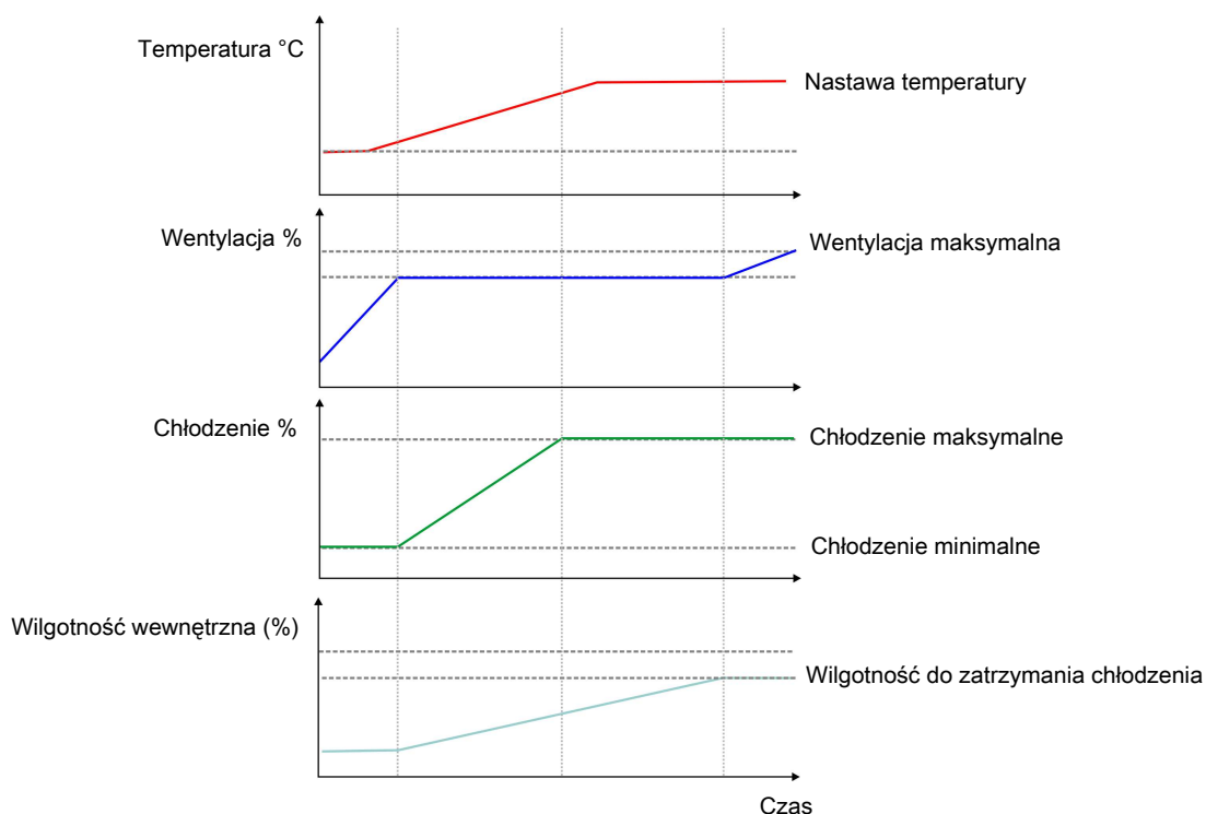
Rysunek 26: Aby utrzymać wymaganą temperaturę wewnętrzną, chłodzenie rozpoczyna się przed osiągnięciem poziomu maksymalnej wentylacji. Gdy system chłodzenia nie może utrzymać temperatury, wentylacja zostaje ponownie zwiększona.
