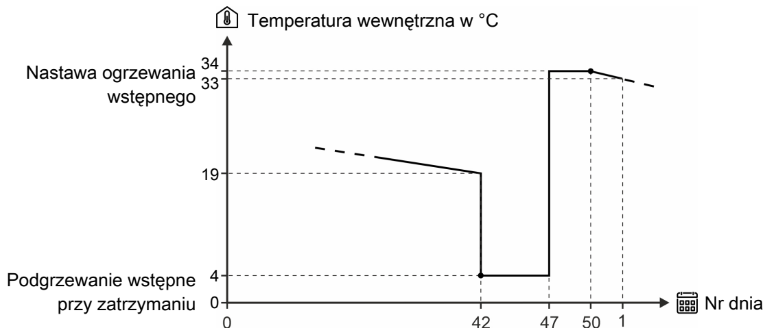
Rysunek 39: Przykładowe ustawienie ogrzewania wstępnego.
