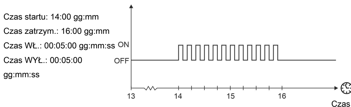
Rysunek 23: Sterowanie zegarem dobowym
