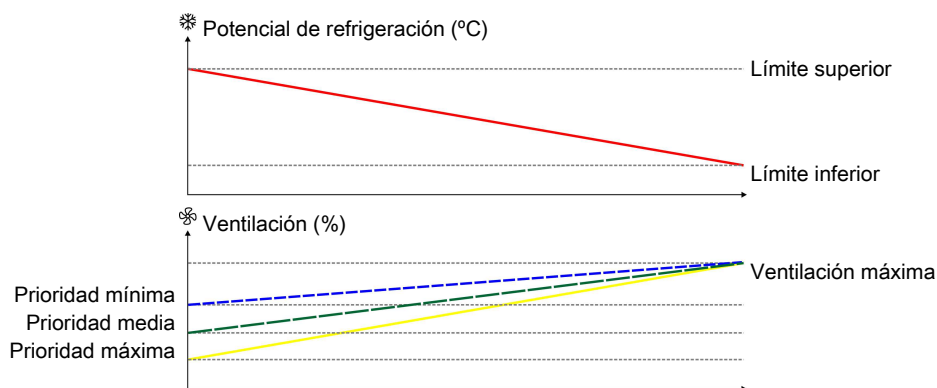
Figura 27: Cuanto mayor sea el potencial de refrigeración, mayor será la prioridad del inicio de refrigeración temprana.
