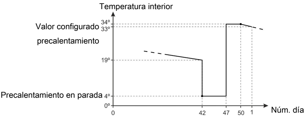
Figura 39: Ejemplo de ajuste de precalentamiento.
