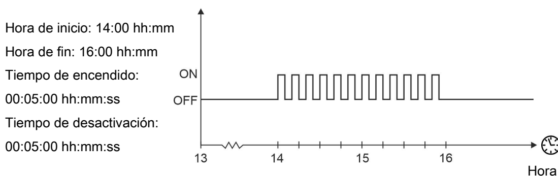
Figura 23: Control reloj 24 horas
