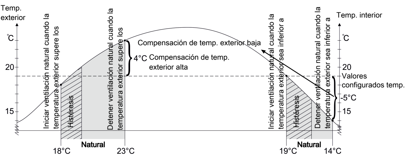
Figura 21: La ventilación natural se encuentra activa en función de la temperatura exterior actual.
