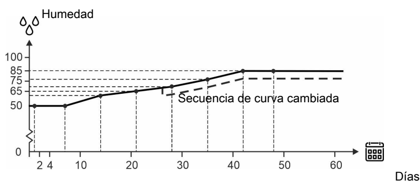
Figura 3: Curva para la humedad del aire
