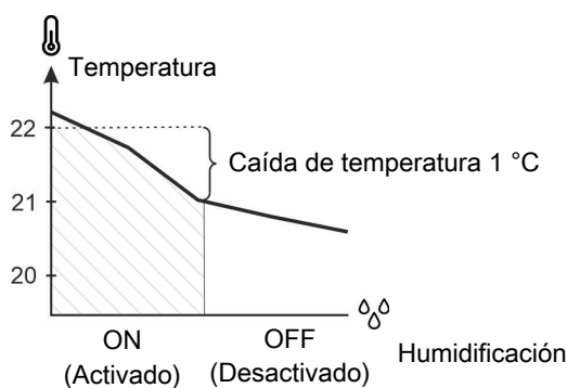
Figura 10: Disminuir la temperatura: La humidificación se desconectará si la temperatura interior está 1 °C por debajo del Valor configurado de temperatura. De lo contrario, la humidificación podría hacer que la temperatura interior descendiera aún más.
