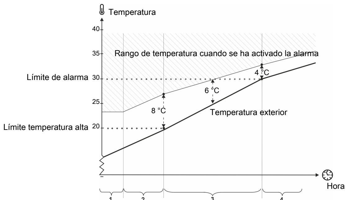
Figura 43: Temperatura de verano a 20 °C y 30 °C en el exterior
