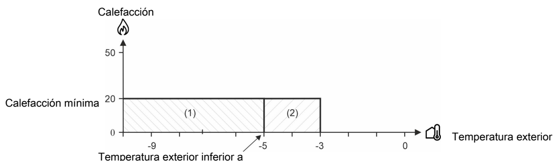
Figura 36: Calefacción mínima al reducirse o incrementarse la temperatura exterior
