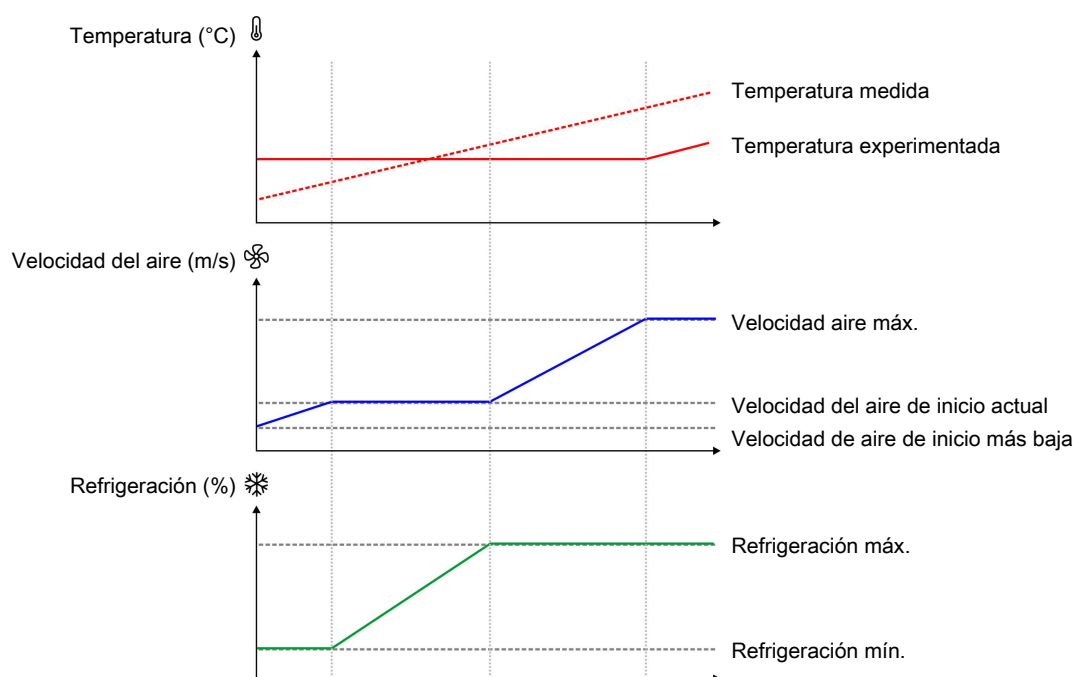
Figura 33: La refrigeración comienza ya a baja velocidad del aire para mantener la temperatura interior requerida. Cuando la refrigeración no puede mantener la temperatura, la velocidad del aire aumenta nuevamente.
