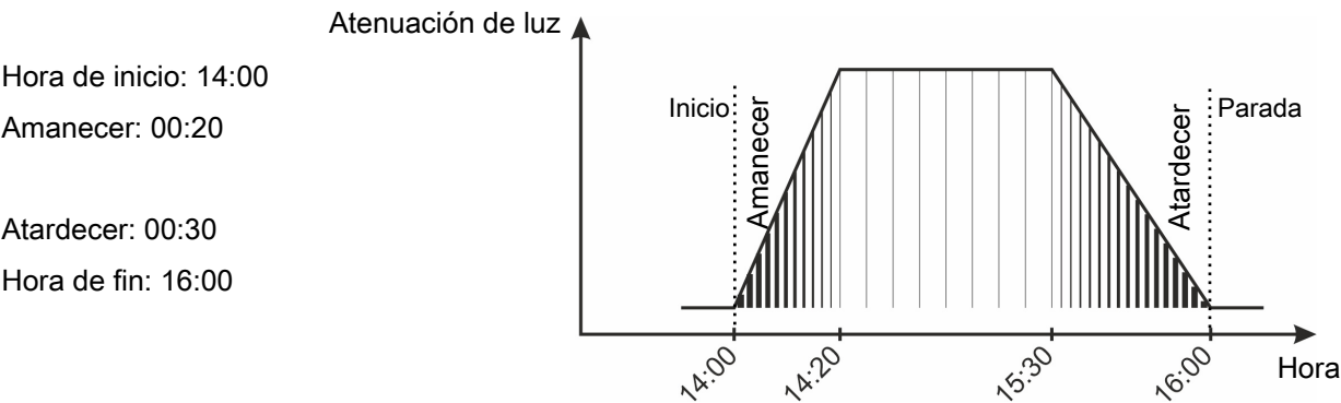
Figura 40: Atenuación de luz normal El amanecer y el atardecer se integran en el periodo de luz.
