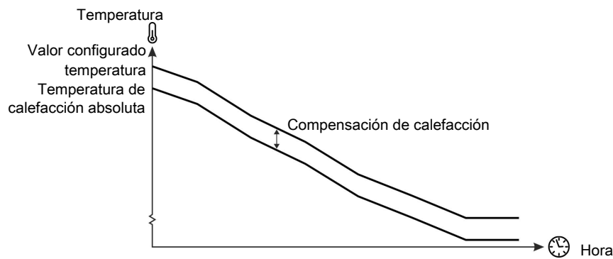
Figura 34: Establecer compensación de calefacción
