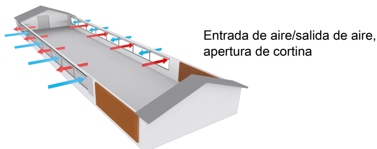
Figura 18: Ejemplo de una nave ganadera con ventilación natural en combinación con ventilación de túnel, ventilación natural.
