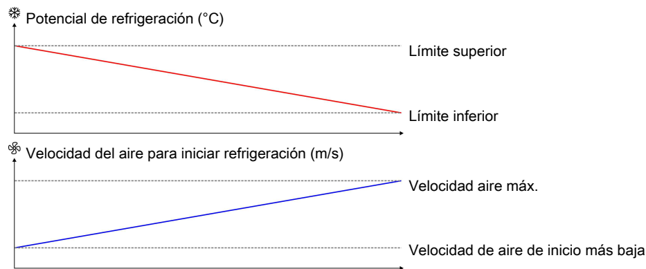
Figura 32: En áreas con baja humedad exterior y un gran potencial de refrigeración, este puede comenzar a una velocidad de aire más baja. Mientras que en áreas con bajo potencial de refrigeración, este comenzará lo más tarde posible, es decir, a la velocidad del aire máxima.
