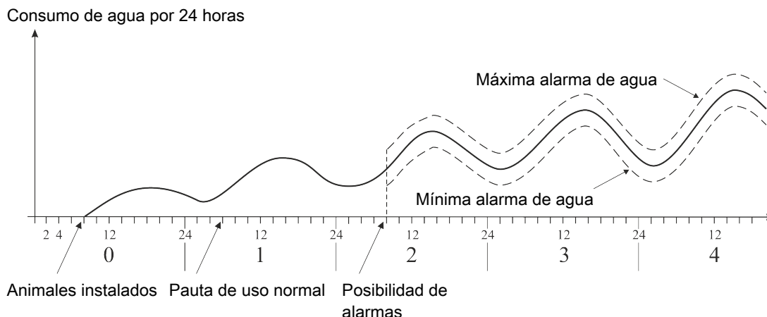
Figura 44: Ejemplo de alarmas de agua mín. y máx.
