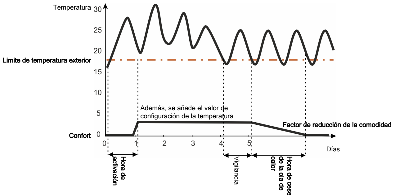
Figura 5: Confort ante ola de calor
