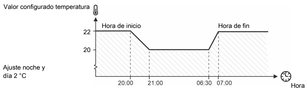
Figura 8: Ajuste de día y noche establecido como un descenso nocturno de la temperatura.
