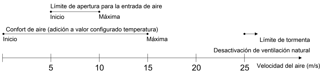
Figura 22: Ventilación natural con velocidad del aire en aumento
