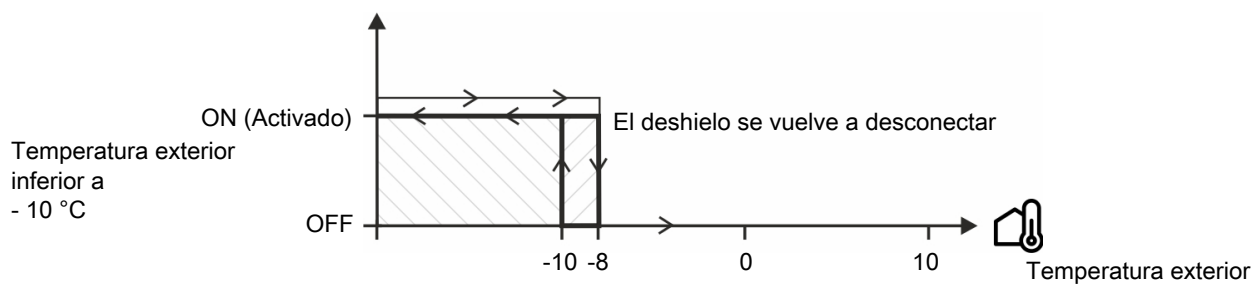
Figura 13: Activación de la función de deshielo
