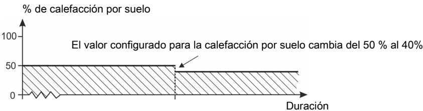
Figura 38: Calefacción por suelo sin sensor de temperatura
