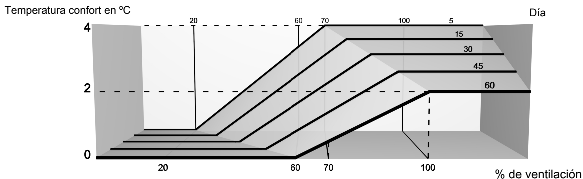
Figura 6: Temperatura confort en producción de lote
