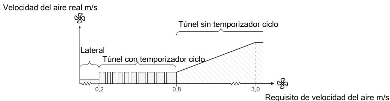
Figura 16: Secuencia de ventilación con temporizador de ciclo en la ventilación de túnel.
