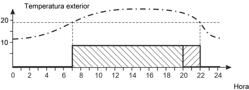
Figura 31: Pulverización según la hora y la temperatura exterior
