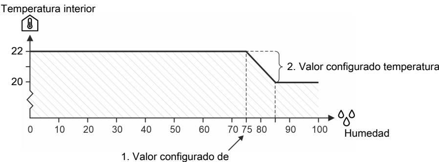
Figura 12: Control de humedad con reducción de temperatura El controlador de la nave disminuirá la temperatura establecida en 1 °C cada vez que la humedad del aire supere el valor configurado de humedad en un 5 %.
