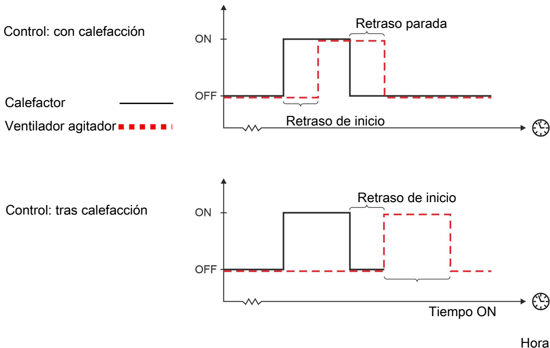
Figura 24: Regulación de la fuente de calor
