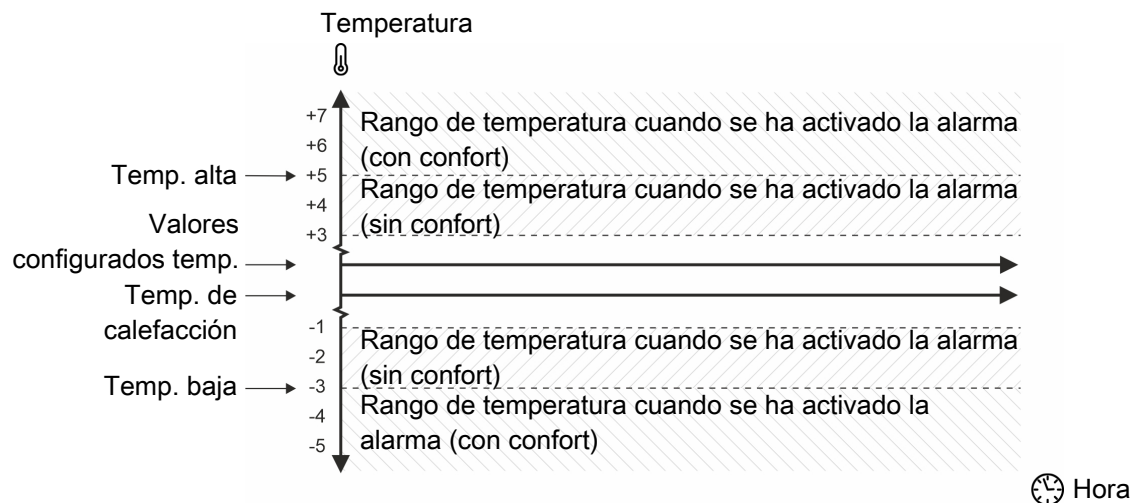
Figura 42: Alarma de temperatura alta y baja
