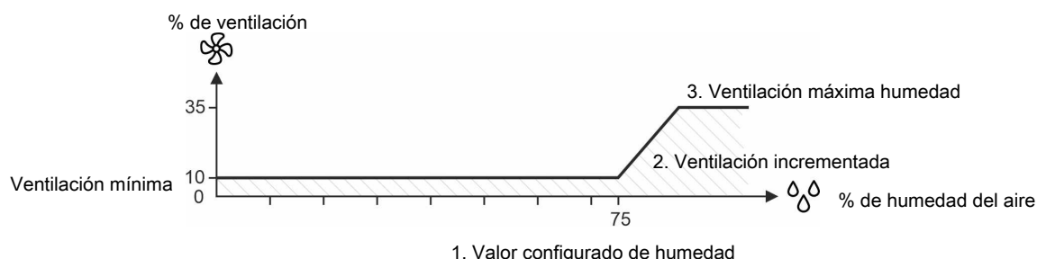
Figura 11: Ventilación de la humedad: 1. La humedad del aire supera el valor configurado de humedad. 2. El controlador aumenta la ventilación. 3. Aumento hasta la ventilación de humedad máxima (35 %).
