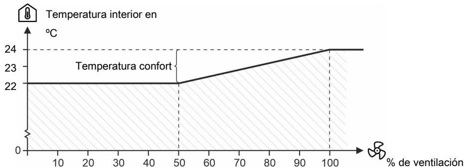
Figura 7: Temperatura confort en producción continua
