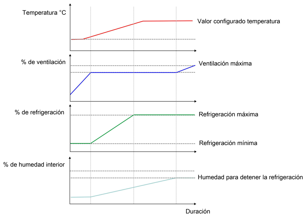
Figura 26: Para mantener la temperatura interior requerida, la refrigeración comenzará antes de que el nivel de ventilación haya alcanzado la ventilación máxima. Cuando la refrigeración no puede mantener la temperatura, la ventilación aumentará nuevamente.
