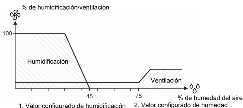
Figura 9: 1. Disminuir la humedad del aire. La humedad del aire está por debajo del valor configurado de humidificación. El controlador inicia la humidificación. 2. Incrementar la humedad del aire. La humedad del aire está por encima del valor configurado de humedad. El controlador aumenta la ventilación.
