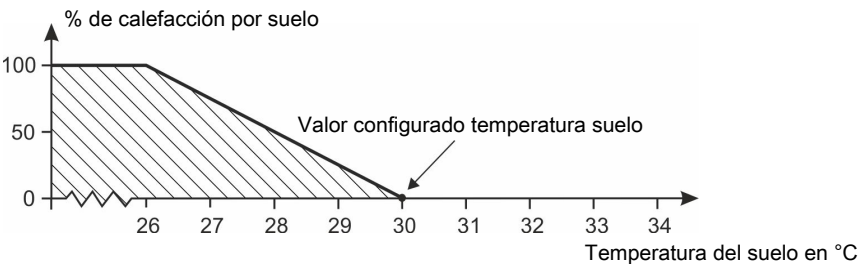
Figura 37: Calefacción por suelo con sensor de temperatura
