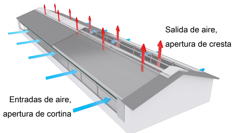
Figura 17: Por ejemplo, una nave con ventilación natural pura, con aperturas de cortina en los laterales y una apertura de cresta en el techo.
