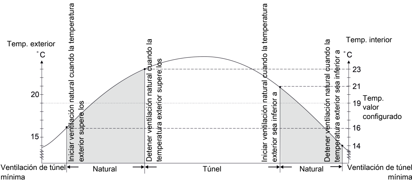
Figura 20: La ventilación natural se encuentra activa en función de la temperatura exterior actual. El valor configurado temperatura es 19 °C.
