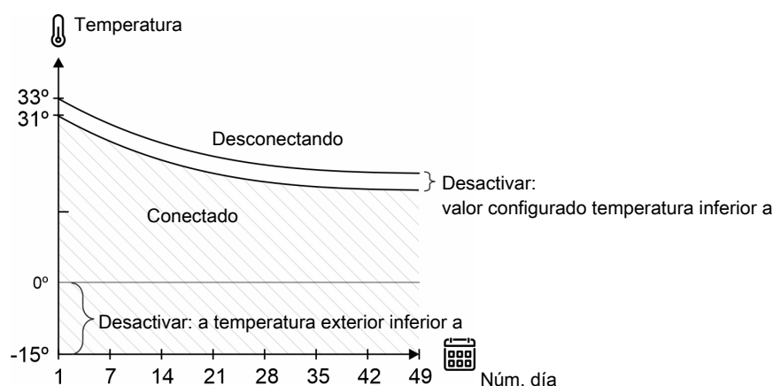
Figura 15: Recuperador de calor: límites temperatura exterior bajos y altos
