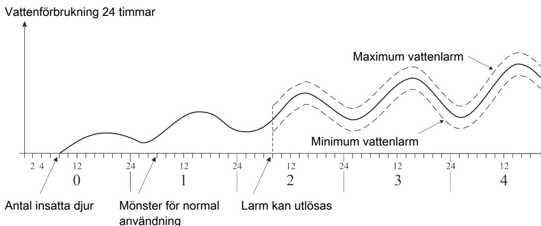
Figur 17: Exempel på minimum och maximum vattenalarm
