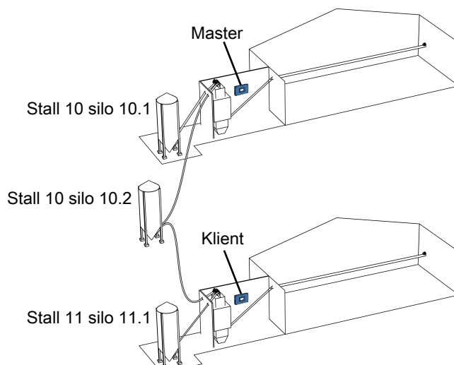
Figur 13: Exempel på silo som delas mellan två stall med styrenheter på LAN-nätet.
