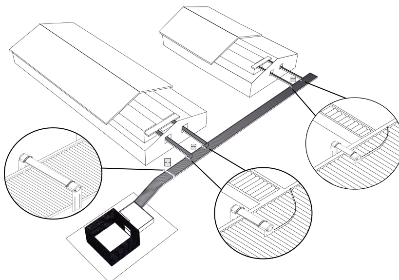
Figur 16: Schematisk ritning över placering av automatisk äggräknare.
