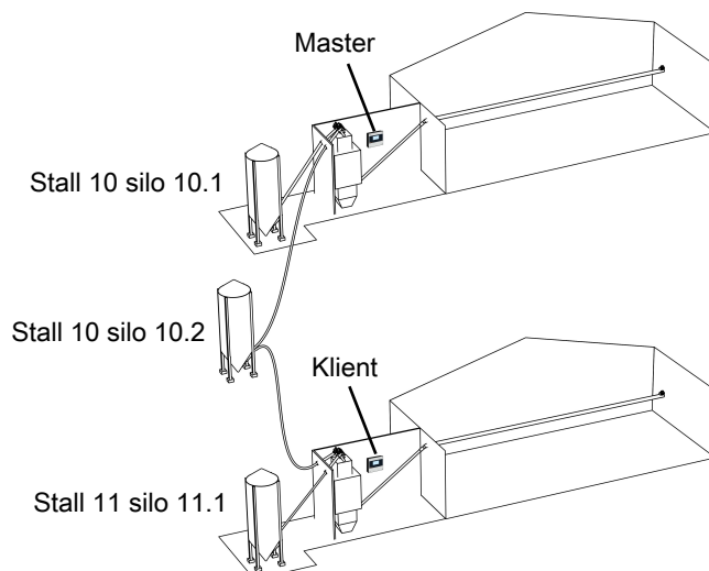
Figur 14: Exempel på silo som delas mellan två stall med styrenheter på LAN-nätet.
