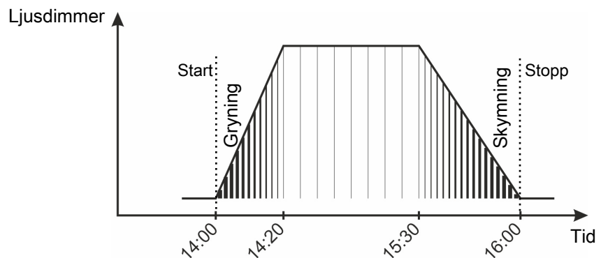
Figur 11: Normal ljusdimmer Gryning och skymning är integrerade i ljusperioden.
