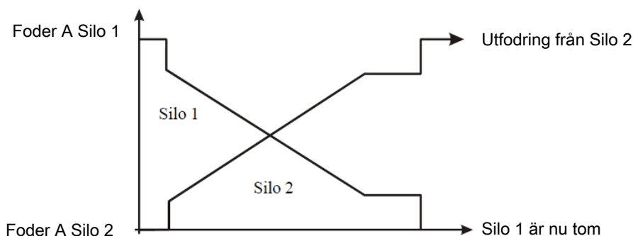
Figur 12: När innehållet i silon når en viss mängd startar den gradvisa övergången till en annan silo.
